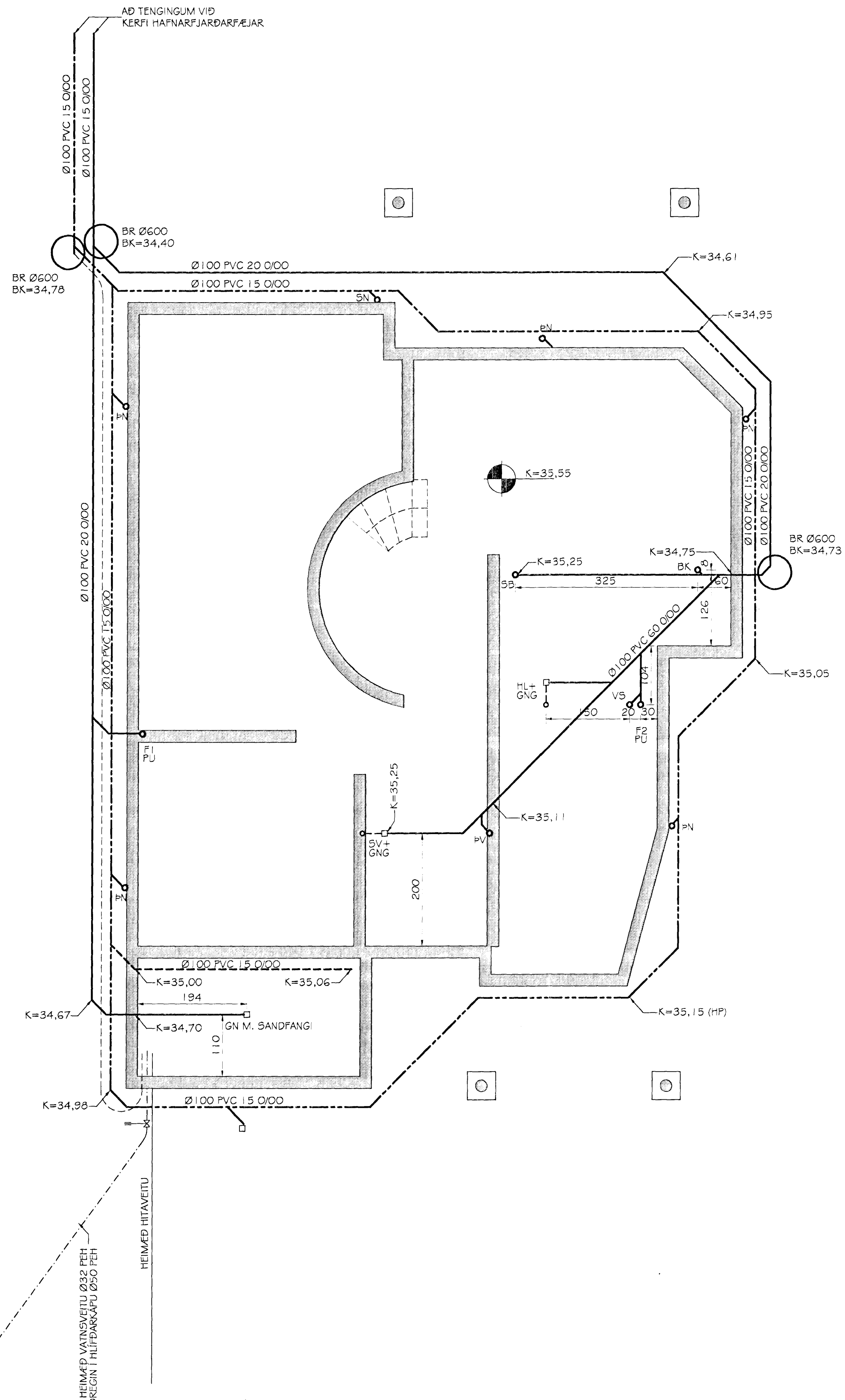
LAGNIR Í JÖRD - GRUNNMYND MKV. 1:50
