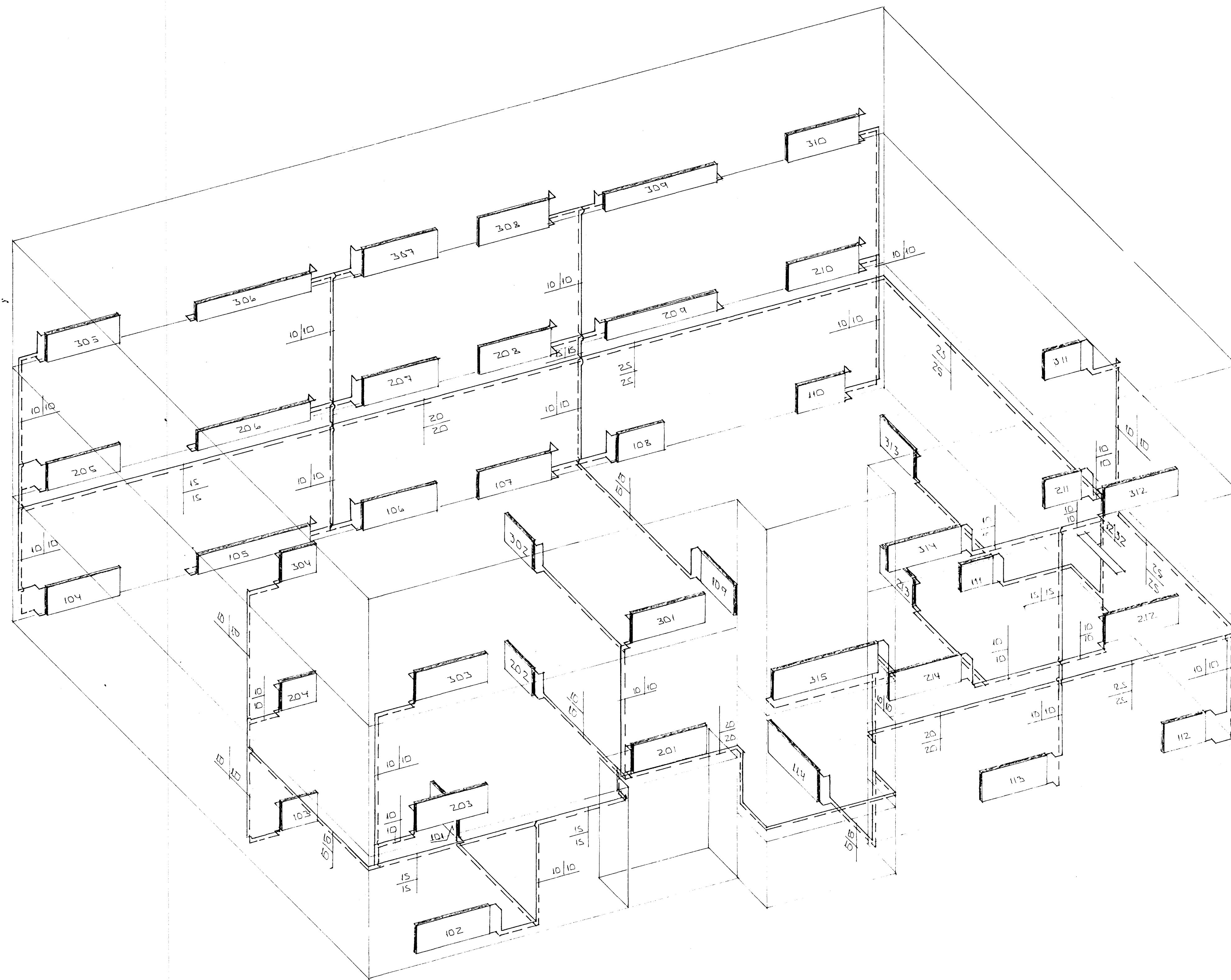
RÚMMYND HITALAGNA 1:50
