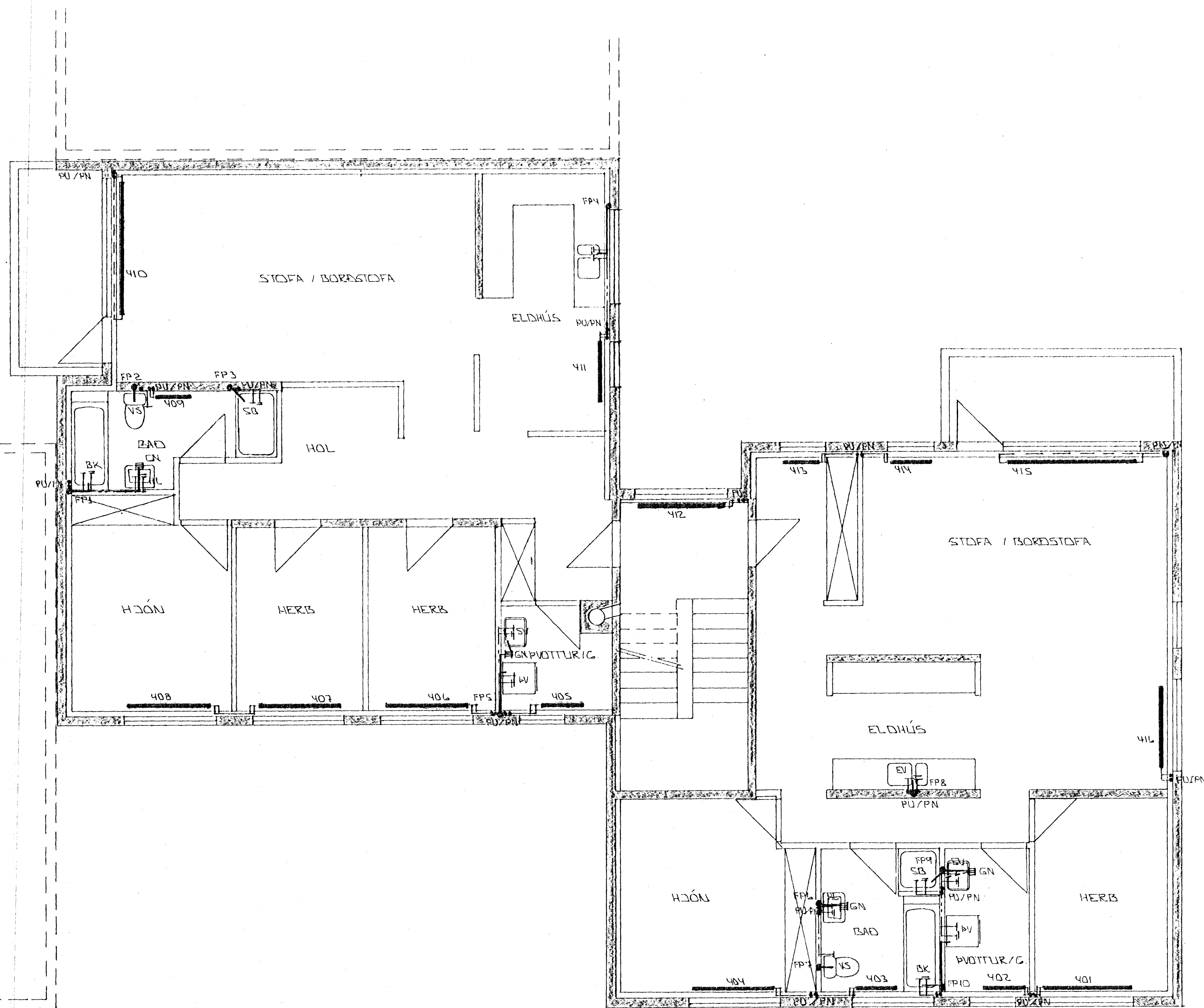
GRUNNMYND 4. HÆÐAR • 1 : 50
