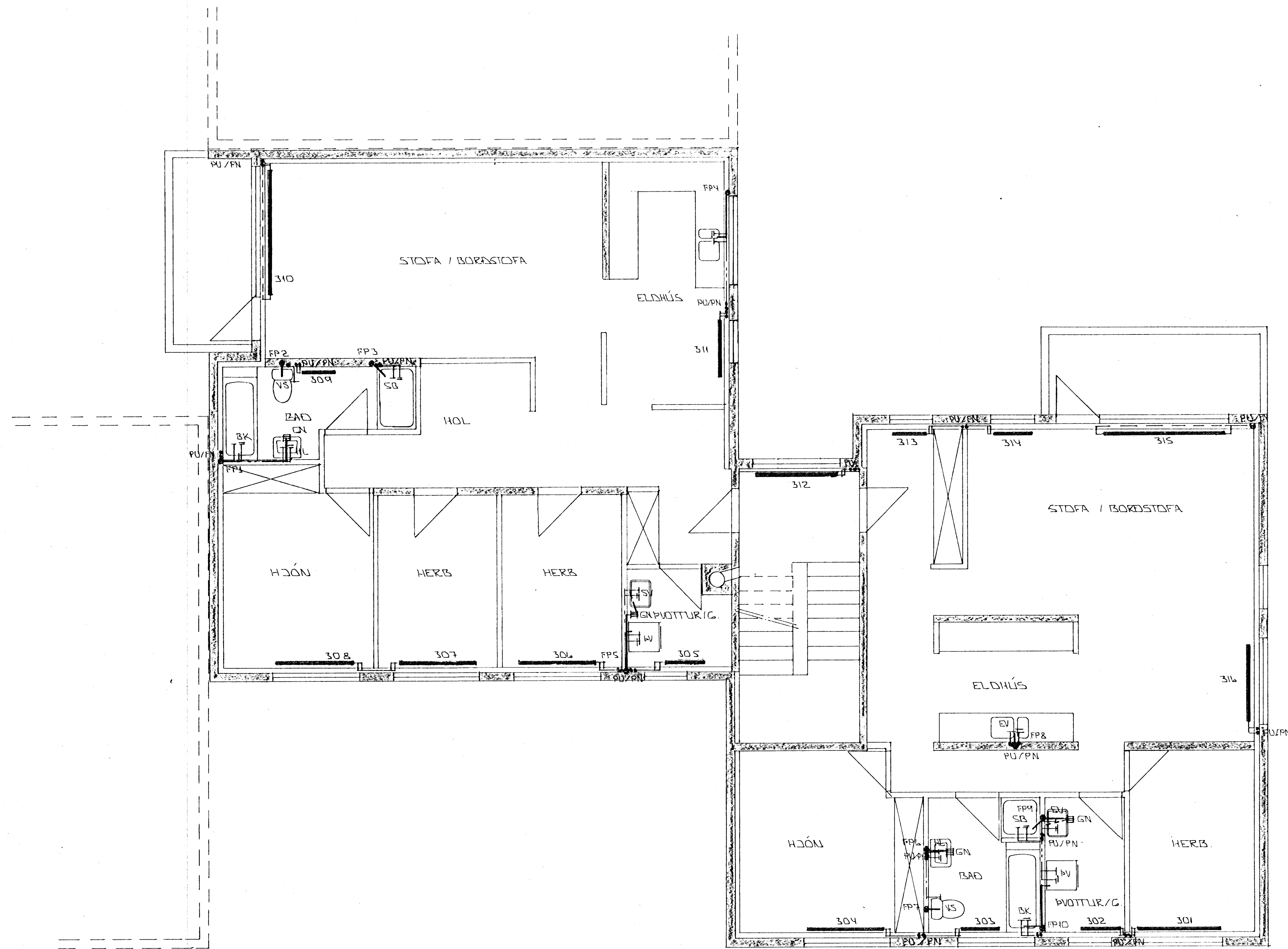
GRUNNMYND 3. HÆÐAR 1:50
