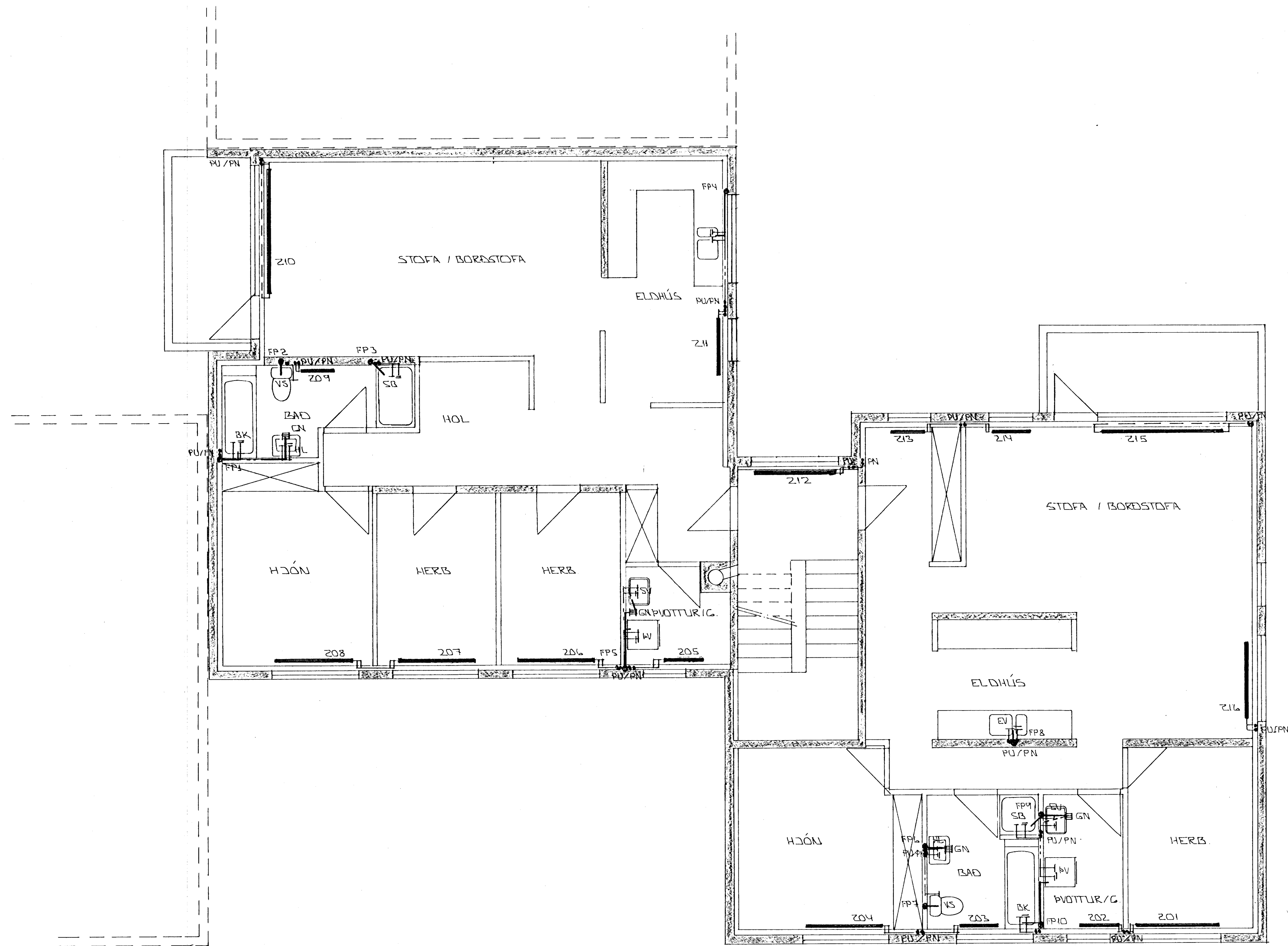
GRUNNMÝND 2. HÆÐAR • 1 : 50
