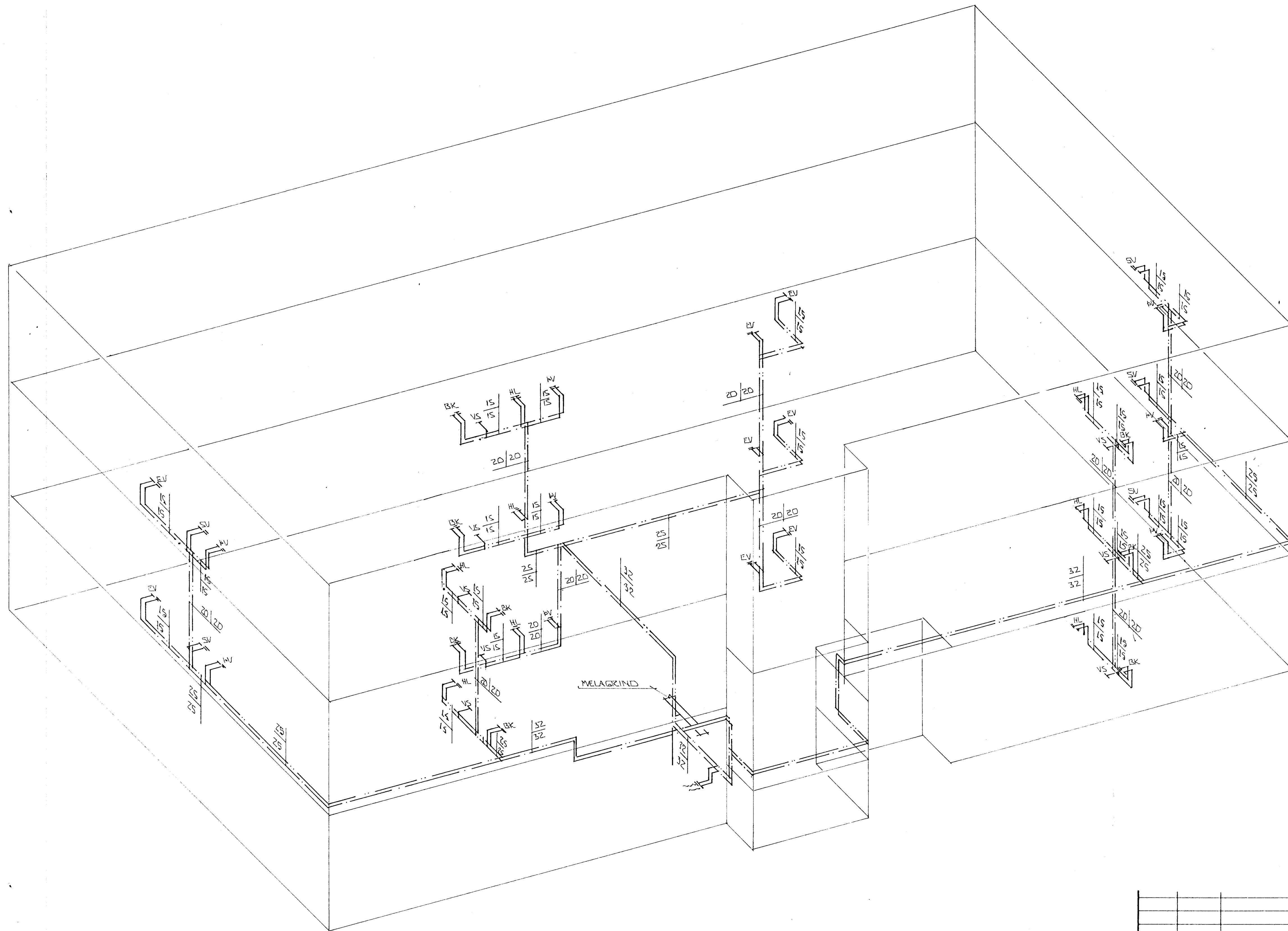
RÜMMYND VATNSLAGNA 1:50
