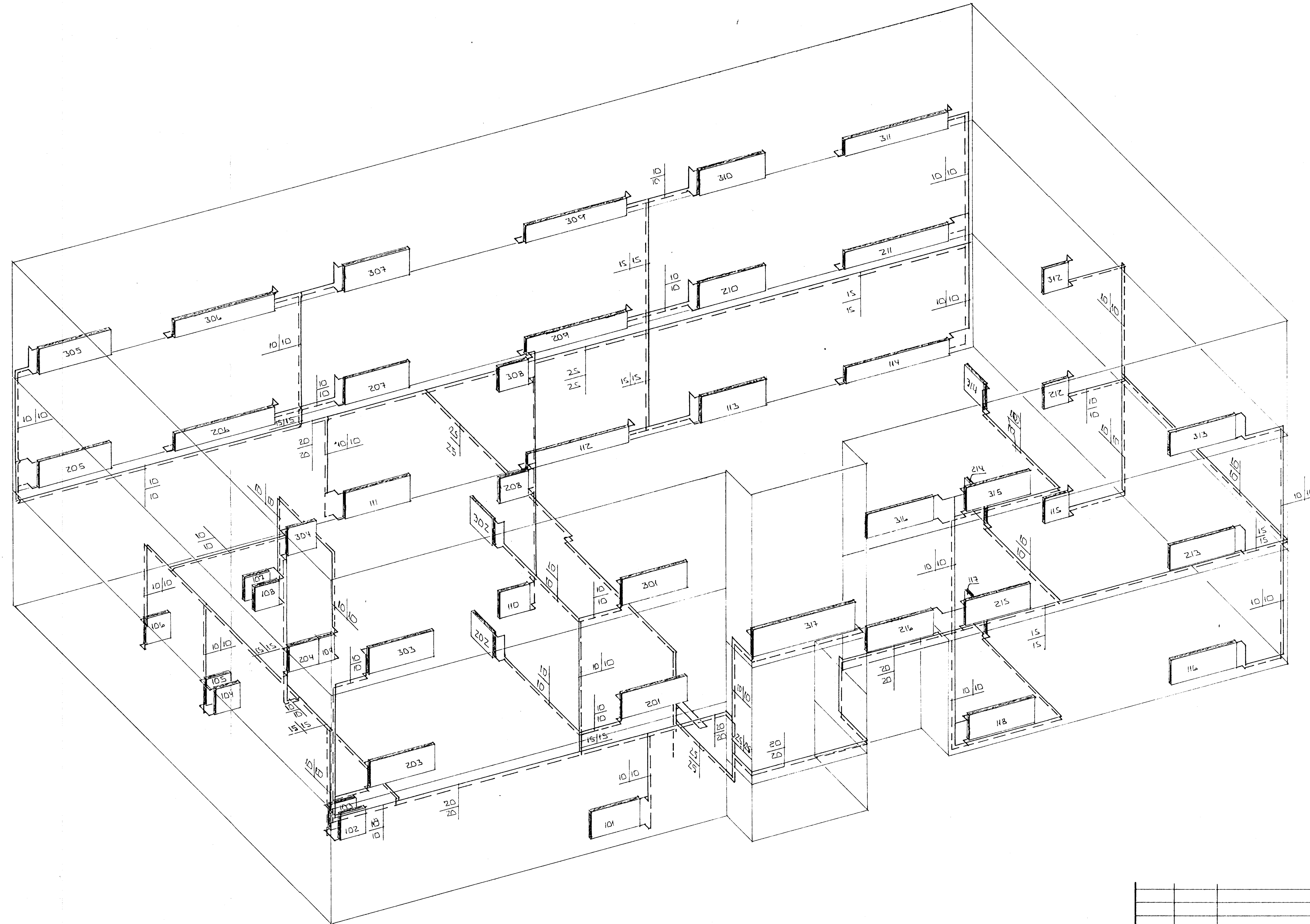
RÚMMYND HITLAGNA 1:50
