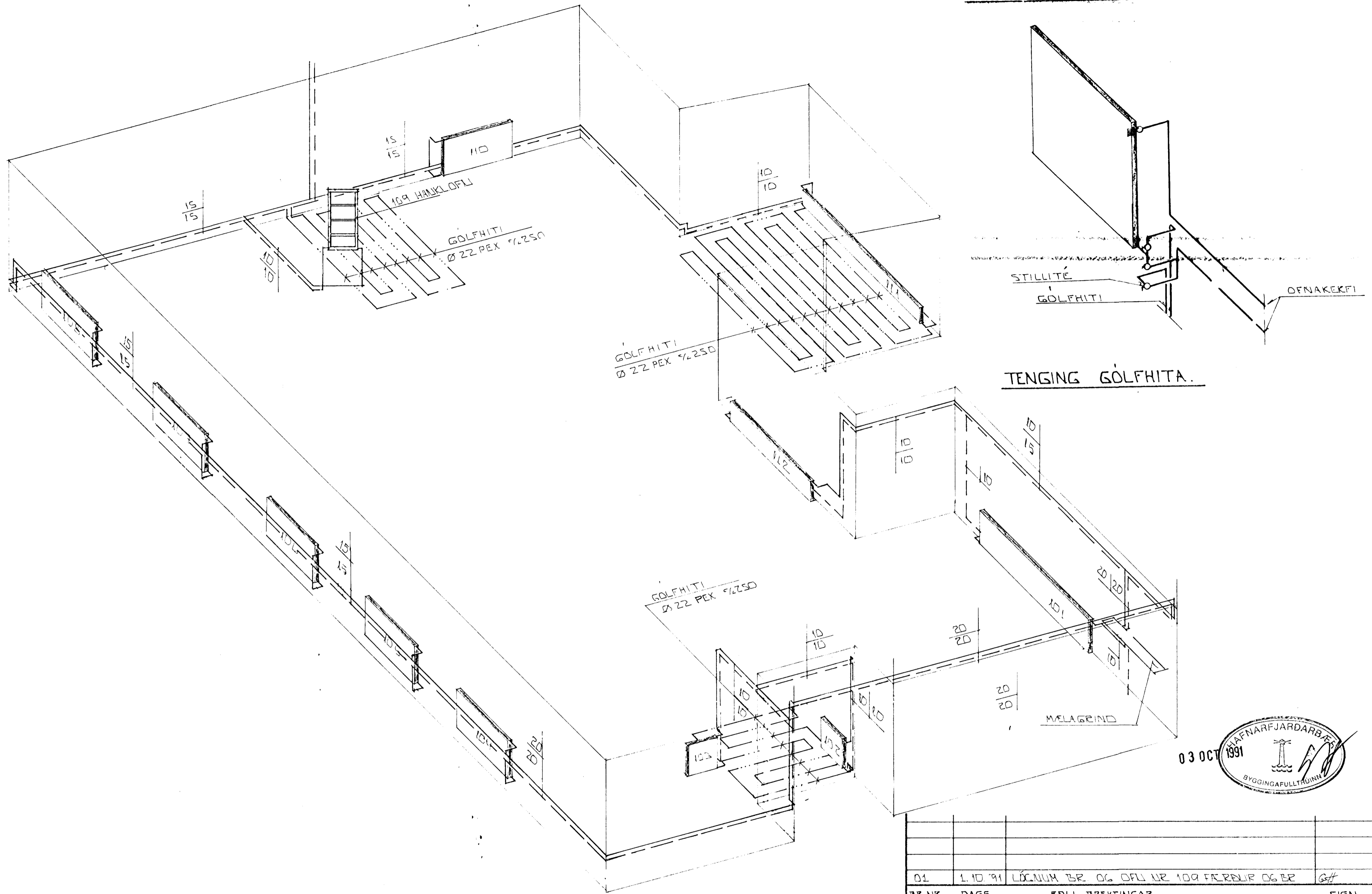
RÜMMYND HITALAGNA · 1:50
