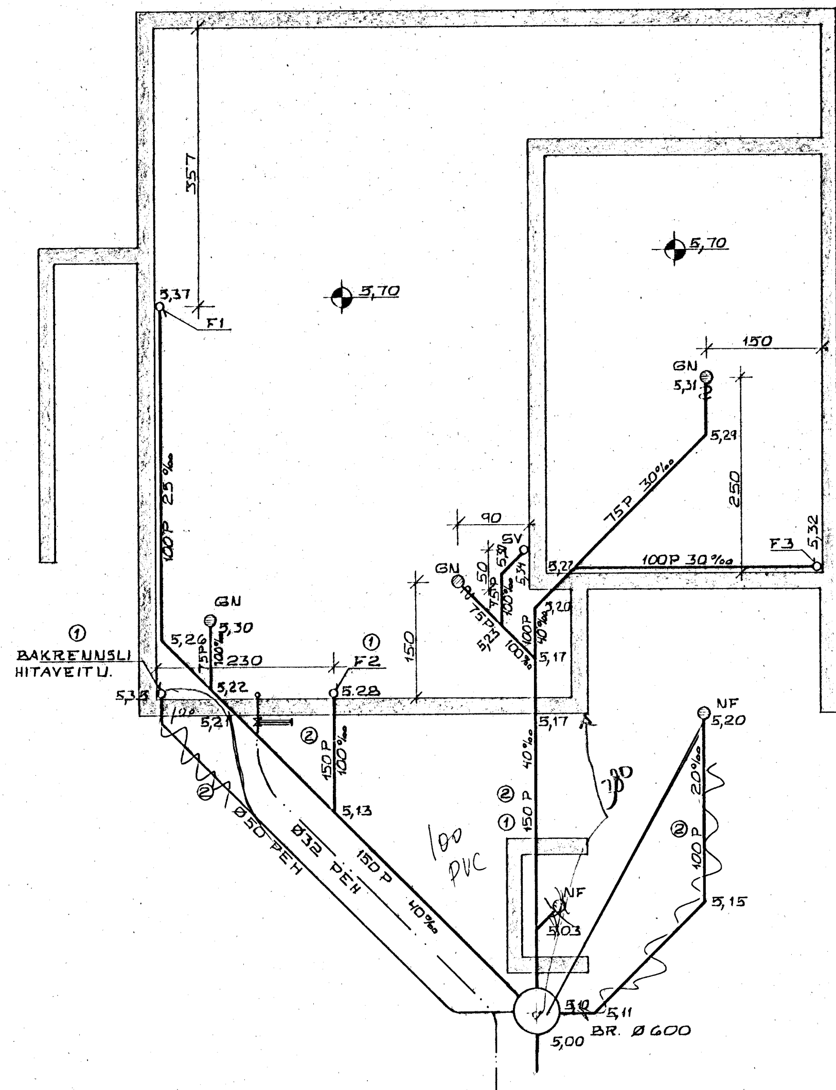
GRUNNMYND 1:50
