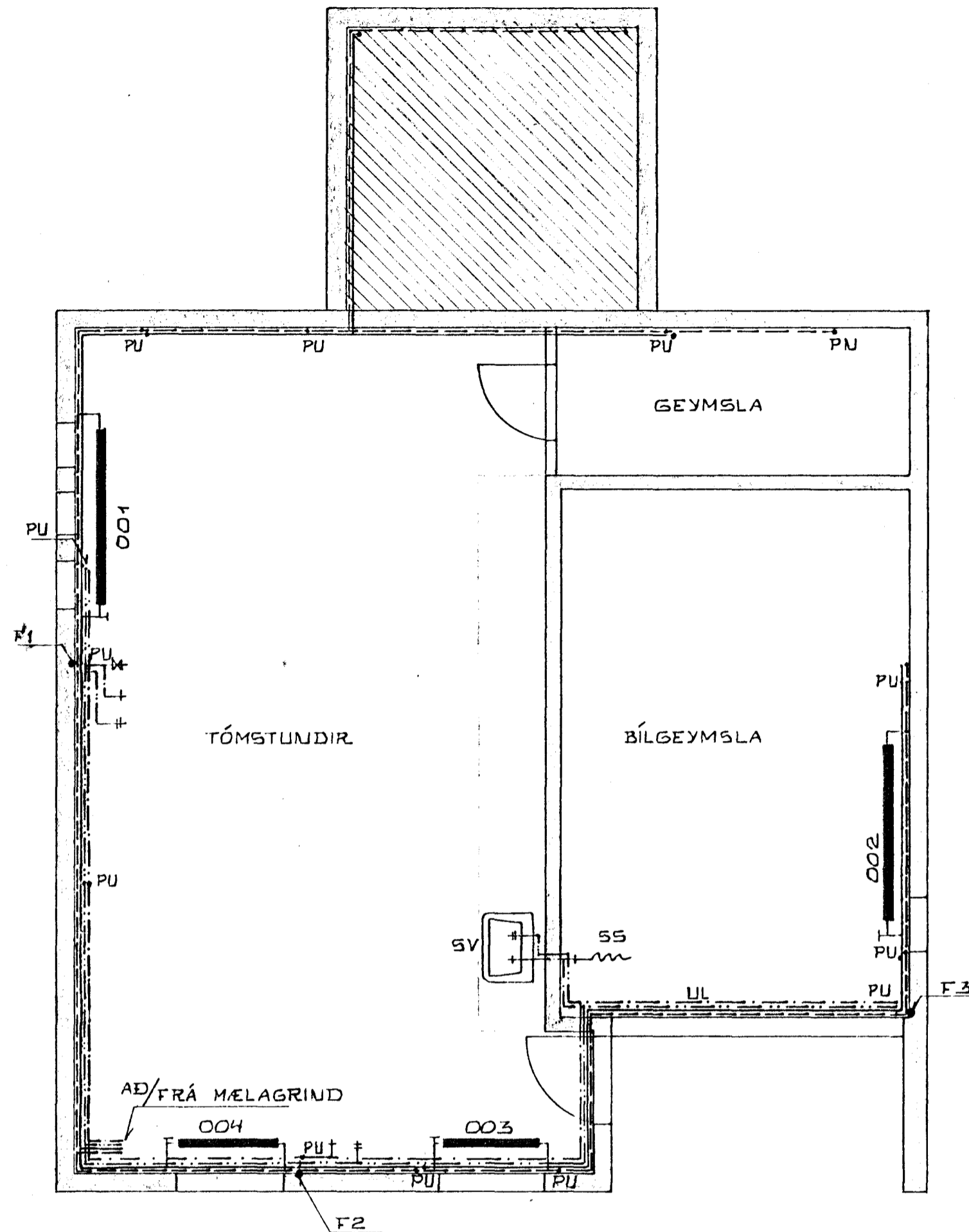
GRUNNMYND KJALLARA 1:50
