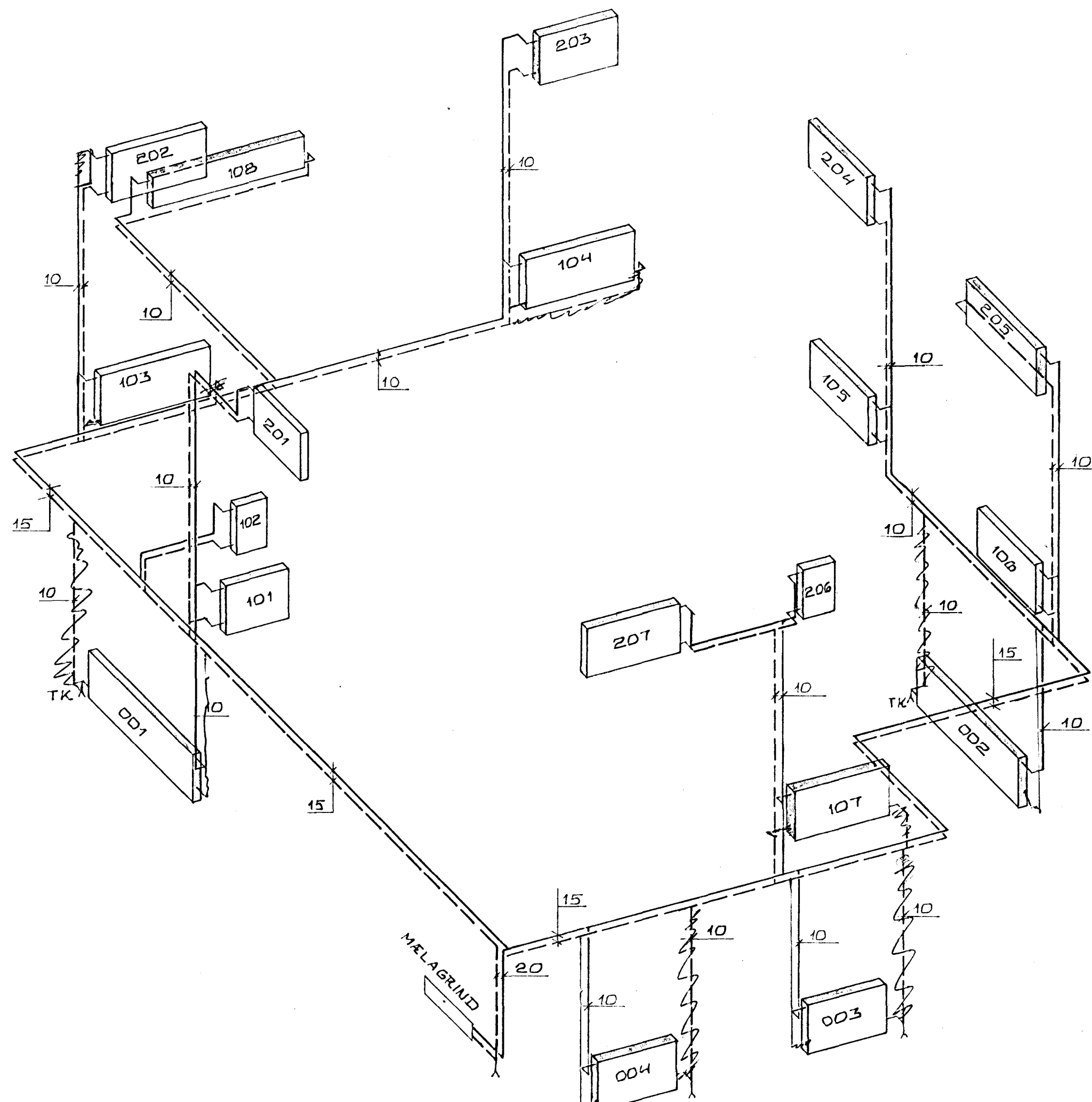
HITALÖGN 1:50
