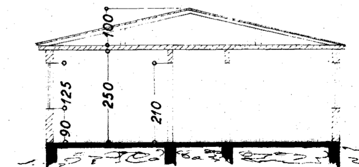
Sneiðing
