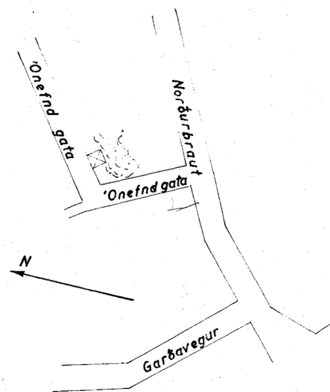
Afstöðumynd 1:2000
