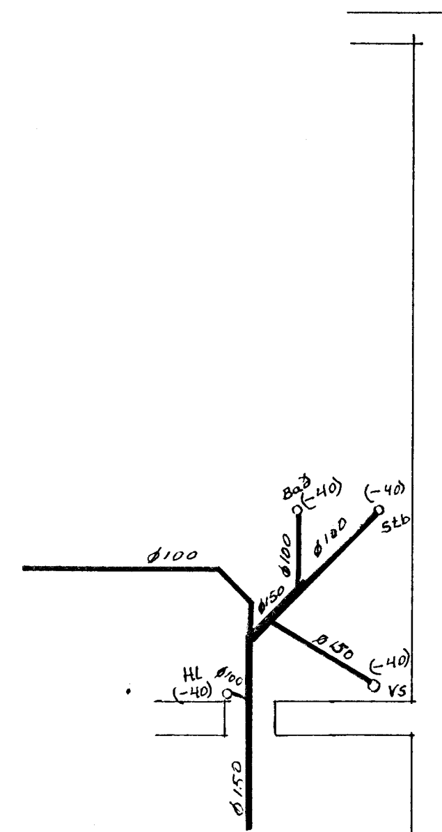
Grunnlögn í bað nr. 31. 1:50
