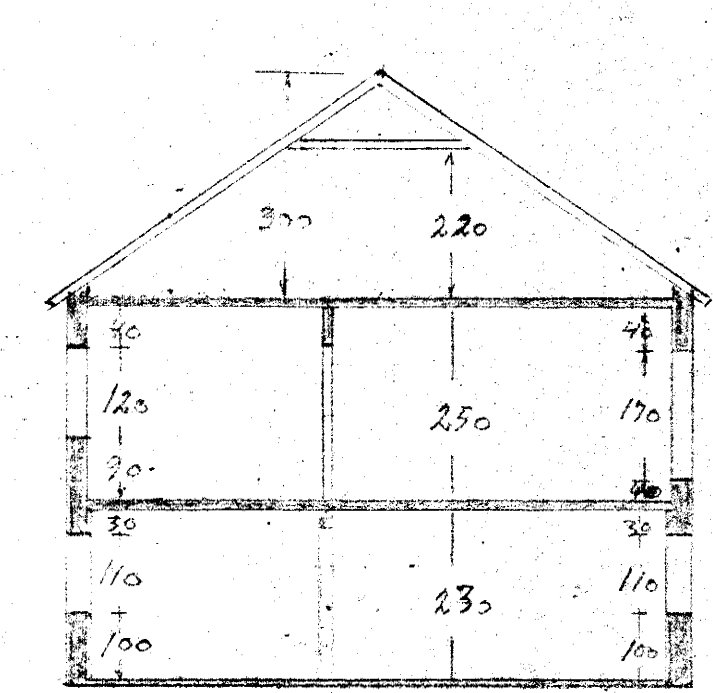
Skurður A-A
