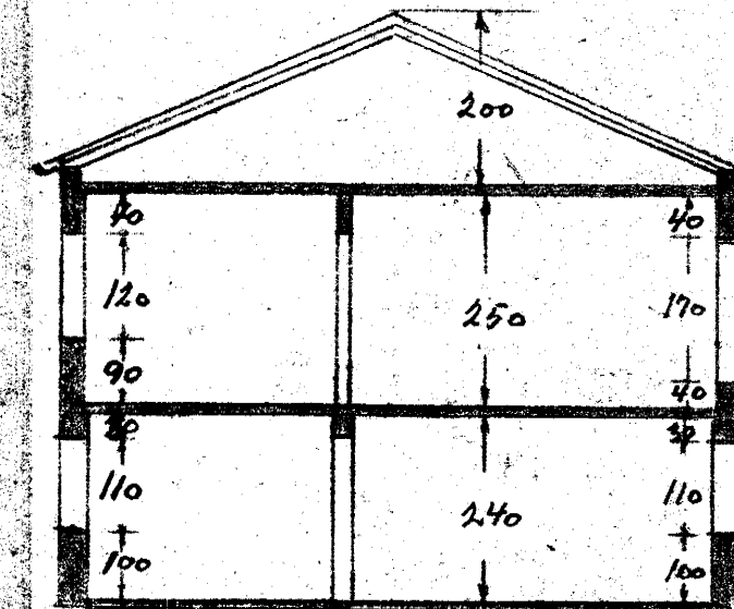
Skurður A-A
