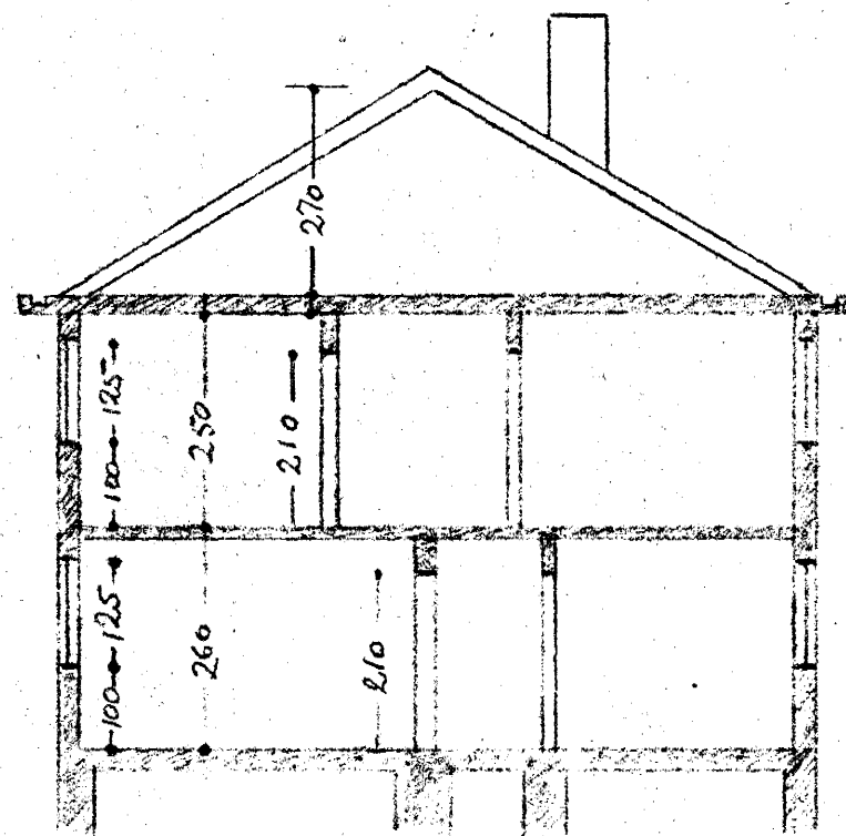
Skurður
