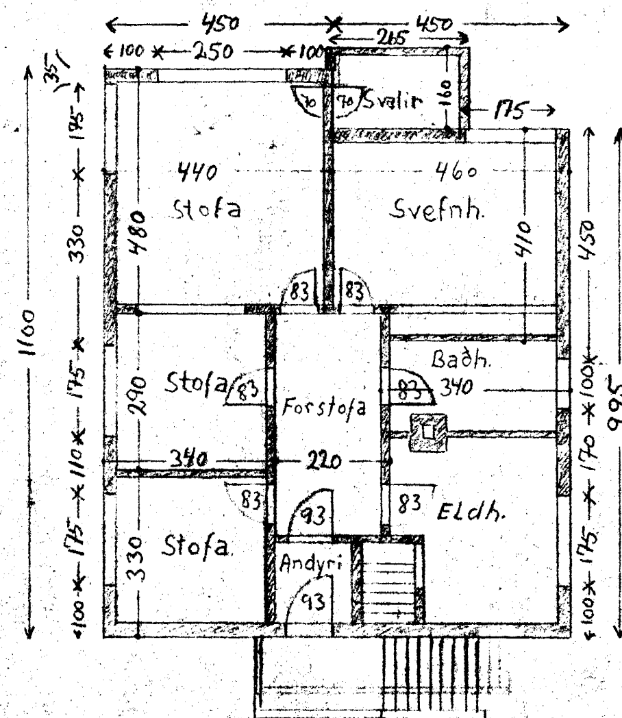
1. hæð
