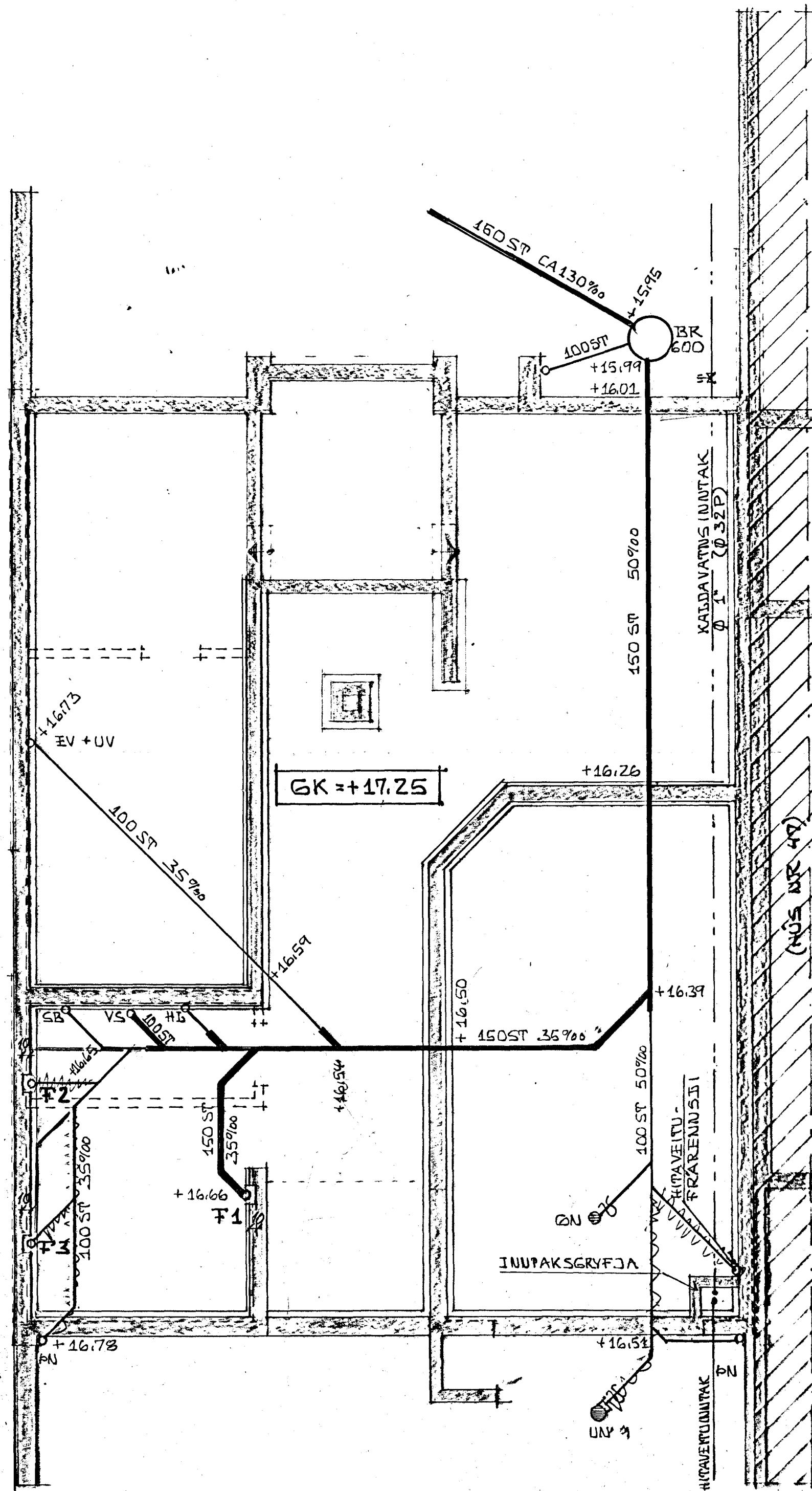
GRUNNMYND 1:50
