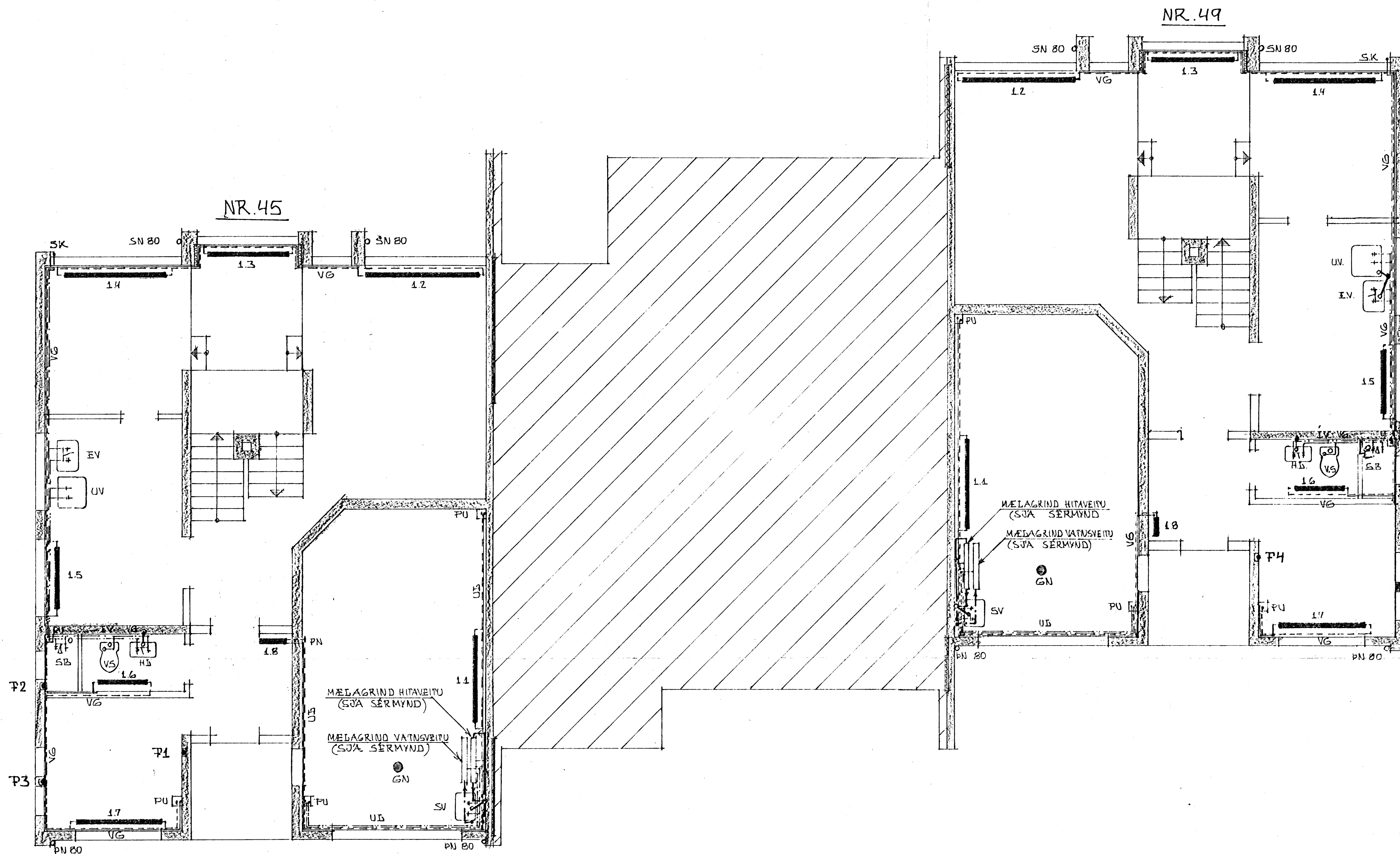
GRUNNMYND 1:50
