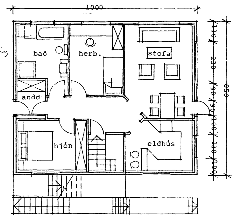
grunnmynd jarðhæðar
