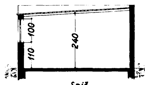
Snið
