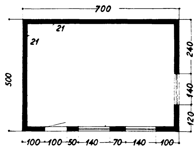
Grunnmynd
