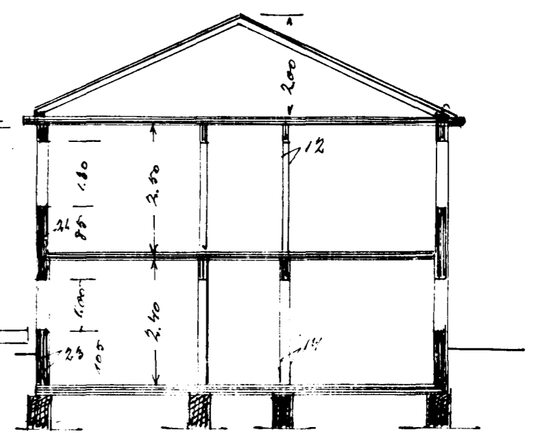
SKIÐULL A-B
