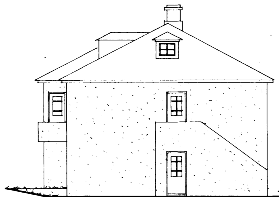
SÚÐUR HLÍÐ
