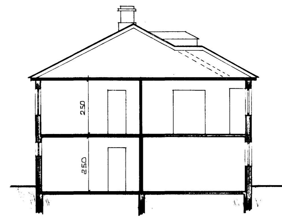
SNEIÐING
