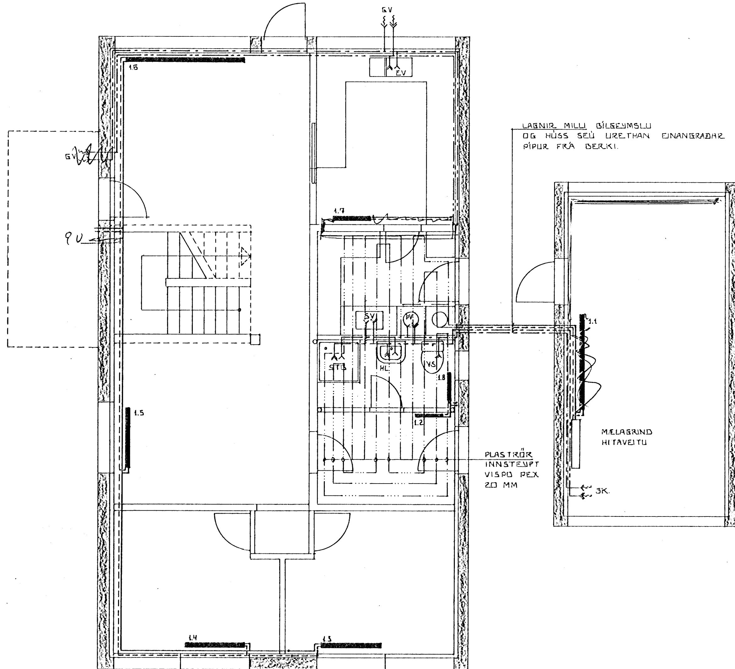
GRUNNMYND 1:50
