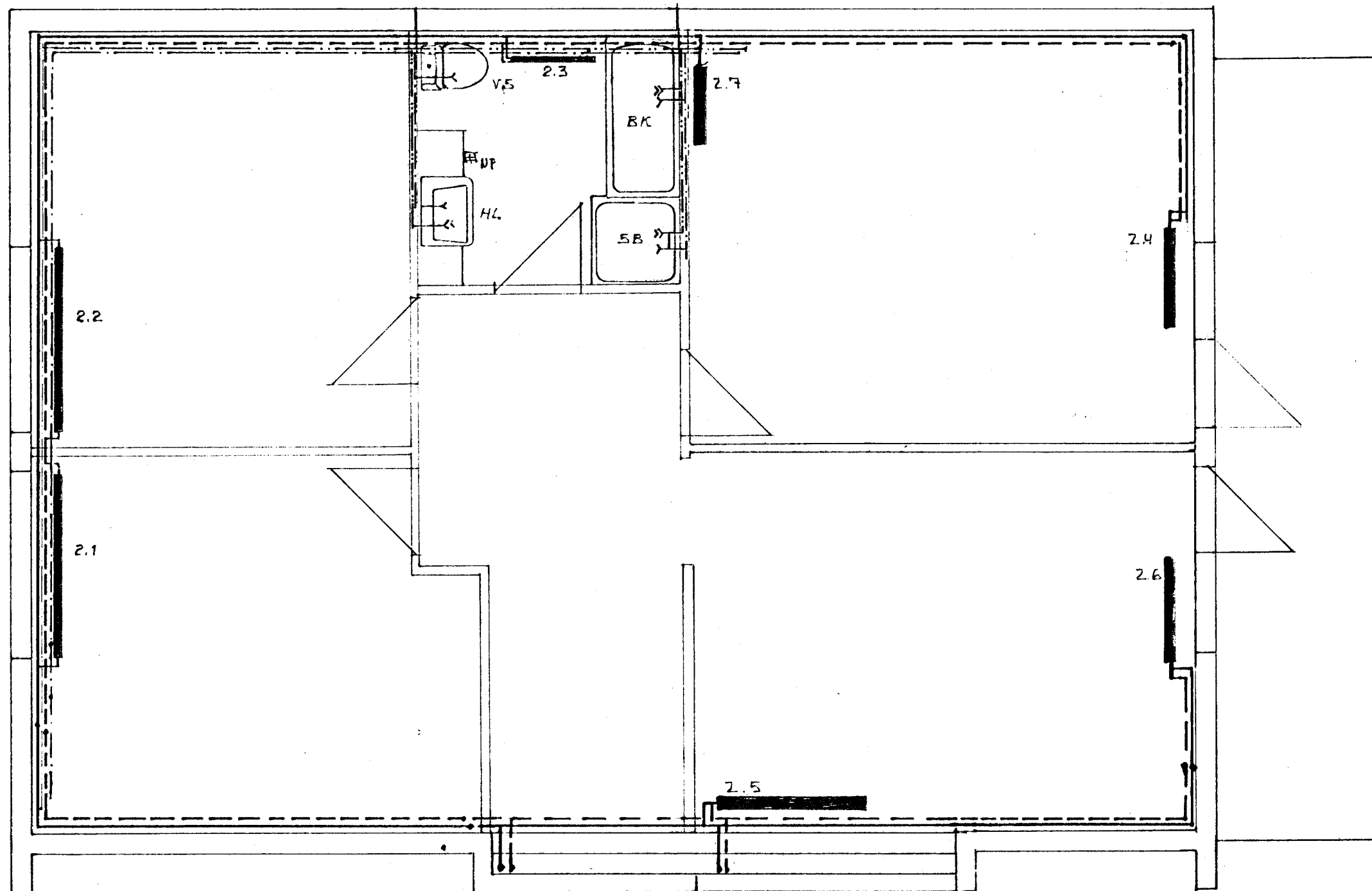
GRUNNMYND RIS 1:50
