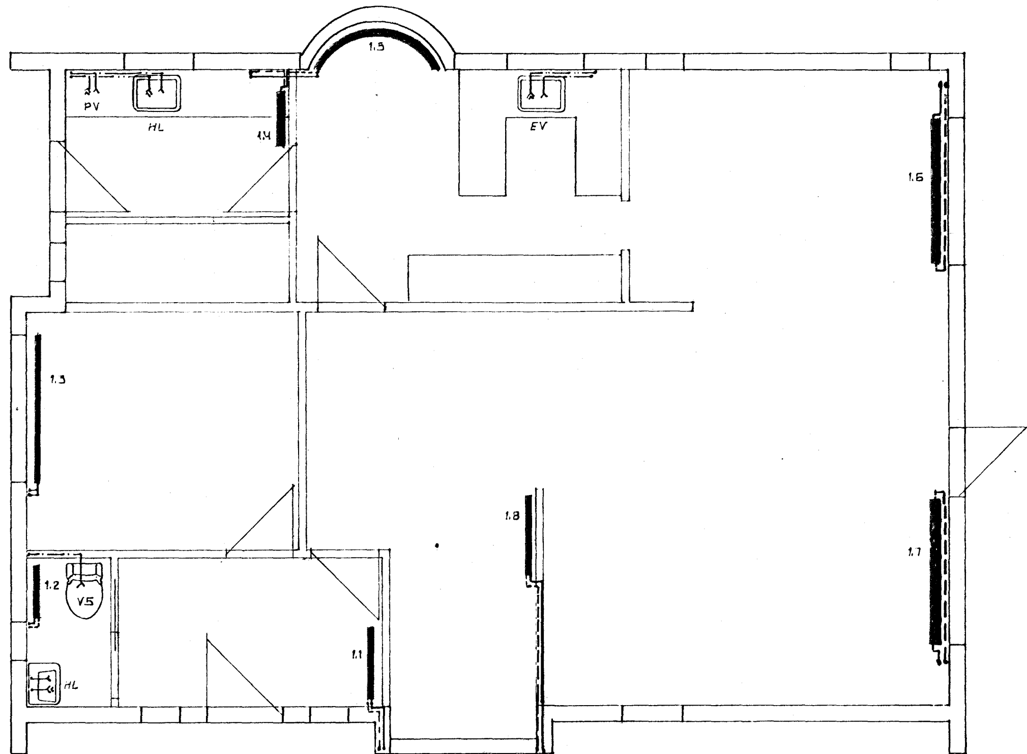
GRUNNMYND HÆÐAR 1:50
