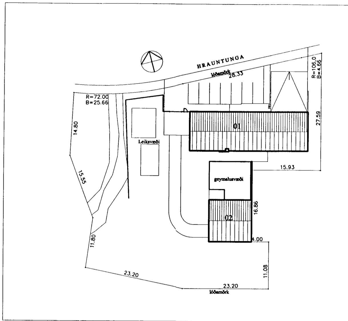
Afstöðumynd 1:500
