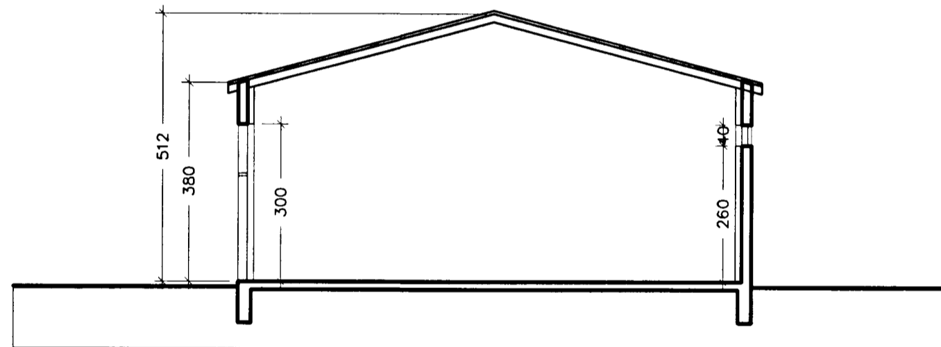
Sneiðing a-a 1:100
