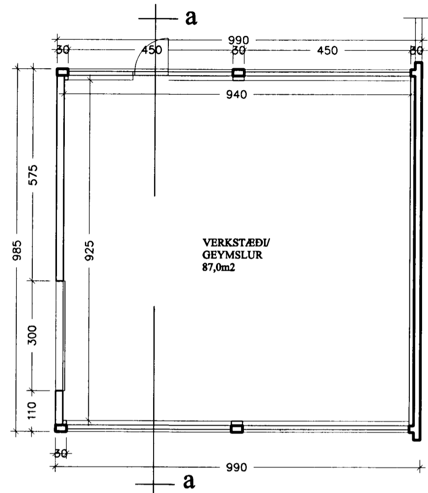
Grunnmynd 1:100
