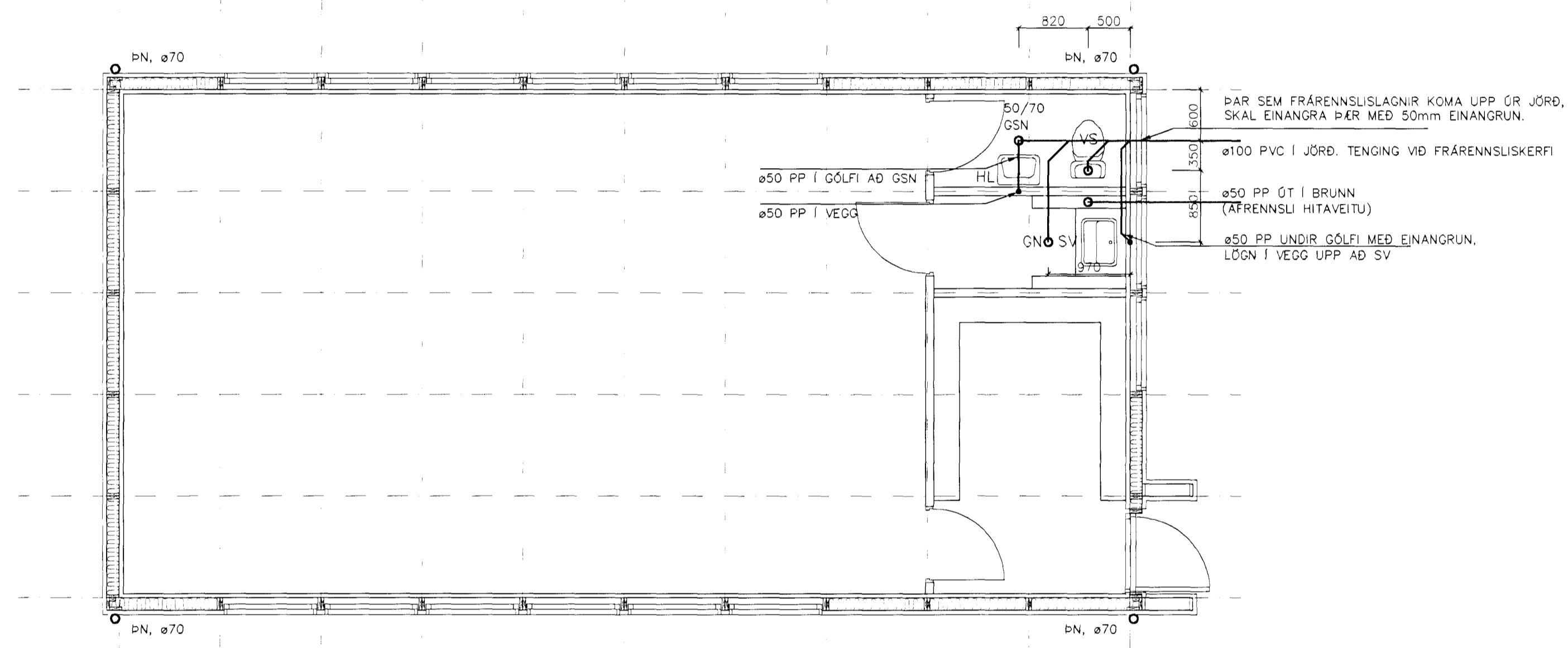
GRUNNMYND FRÁRENNISLAGNA Mkv. 1:50
