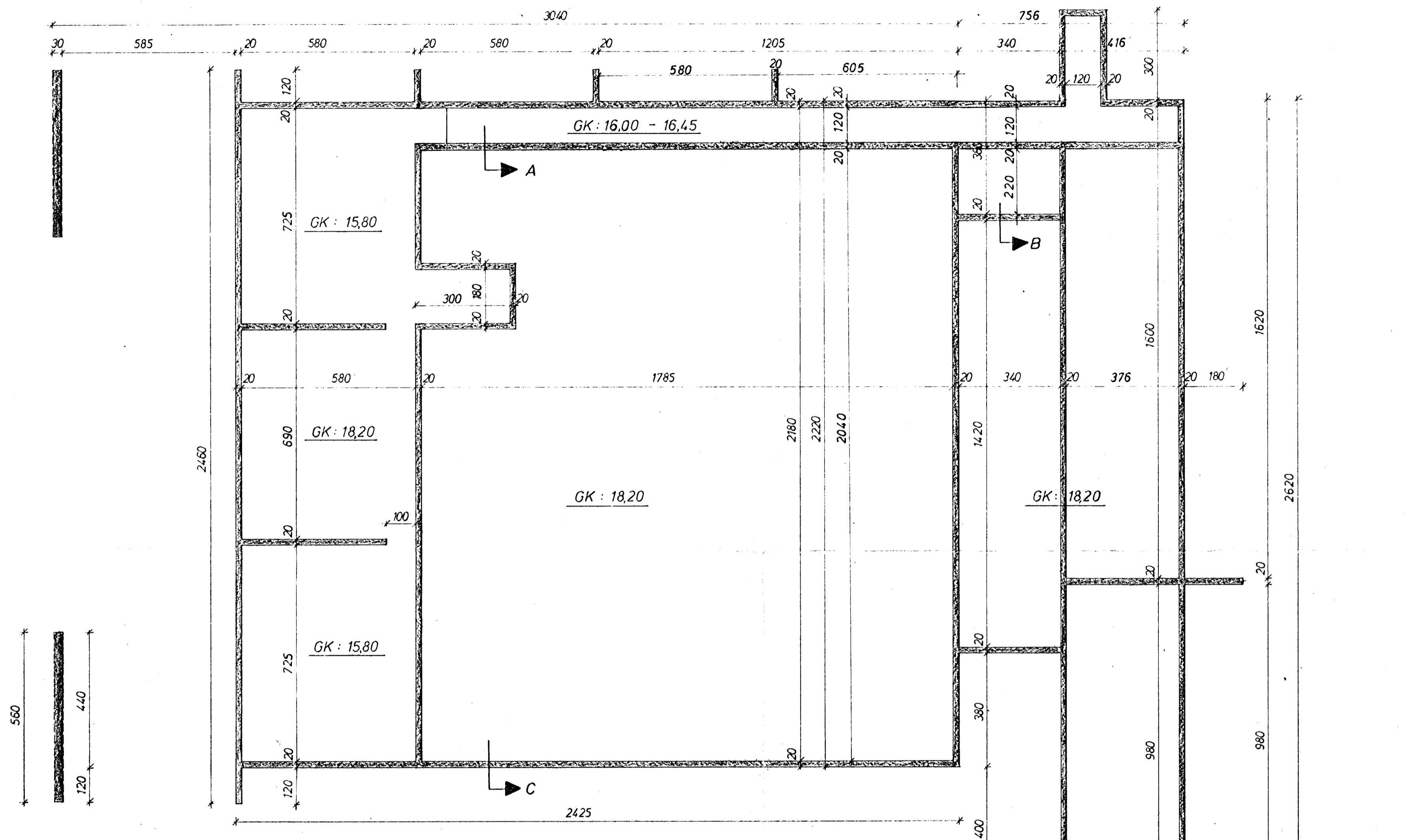
GRUNNMYND 1 : 100
