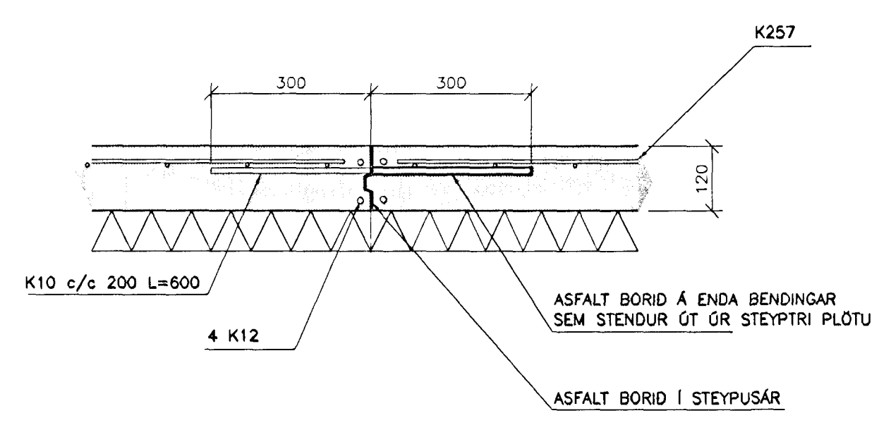
SÉRMYND 1 1:10
