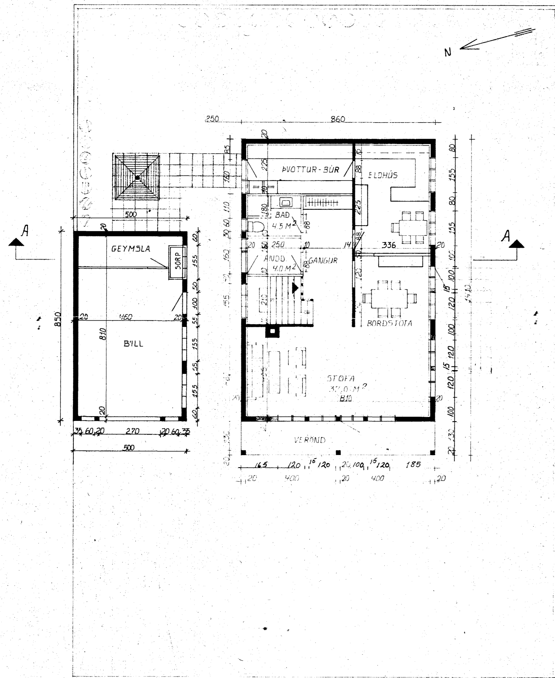
GRUNNMYND HÆÐAR 1:100
