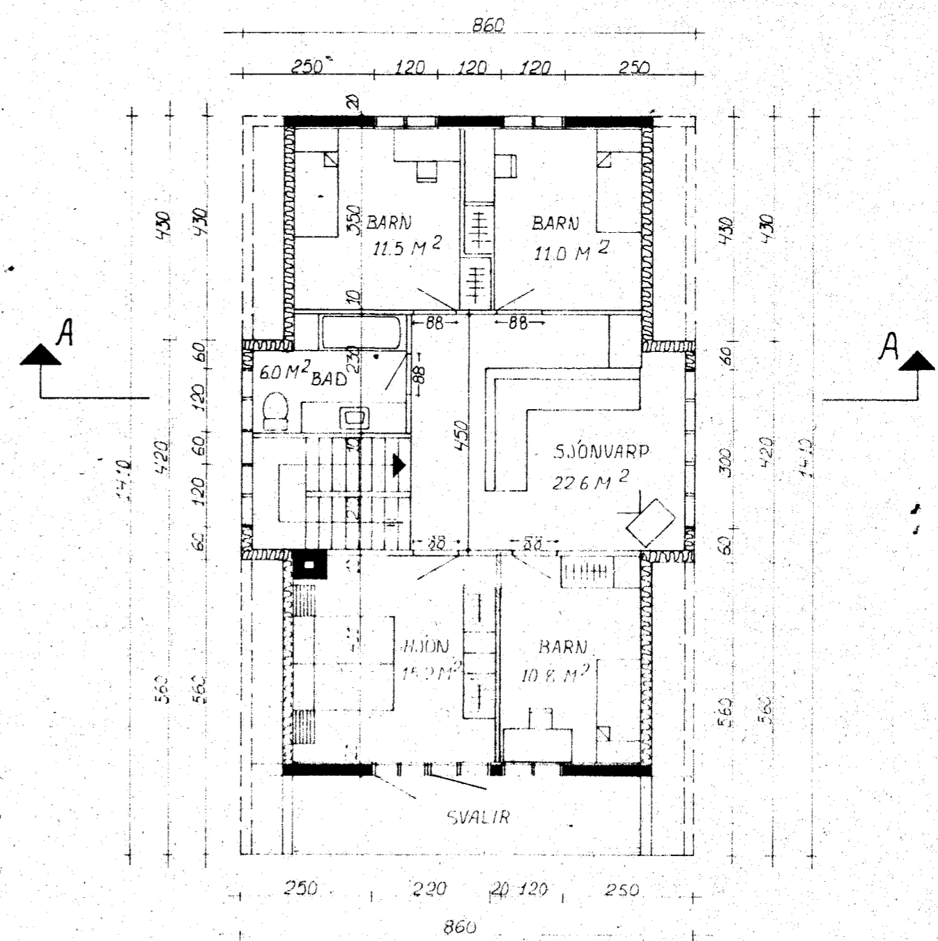
GRUNNMYND RISHÆÐAR 1:100
