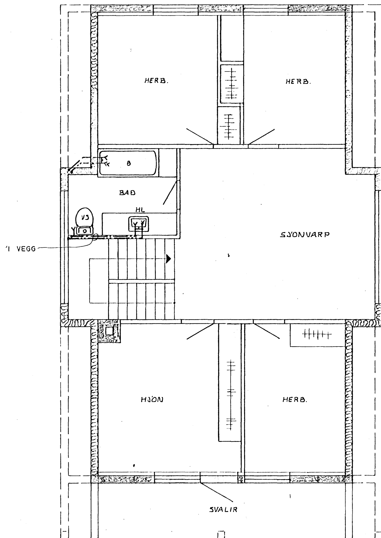
GRUNNMYND - EFRI HÆÐ
