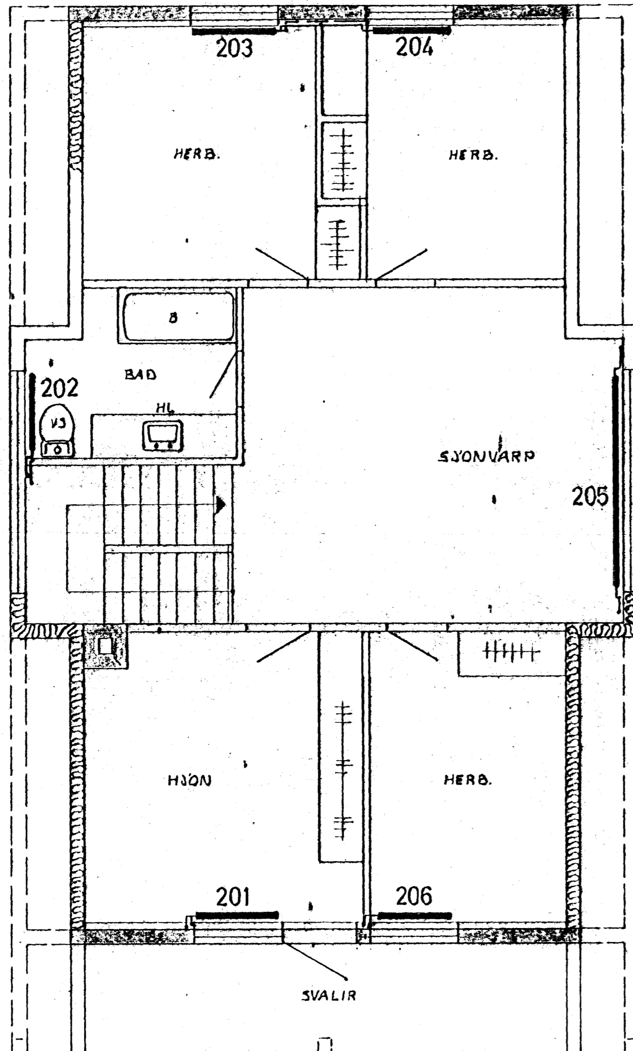
GRUNNMYND - EFRI HÆÐAR
