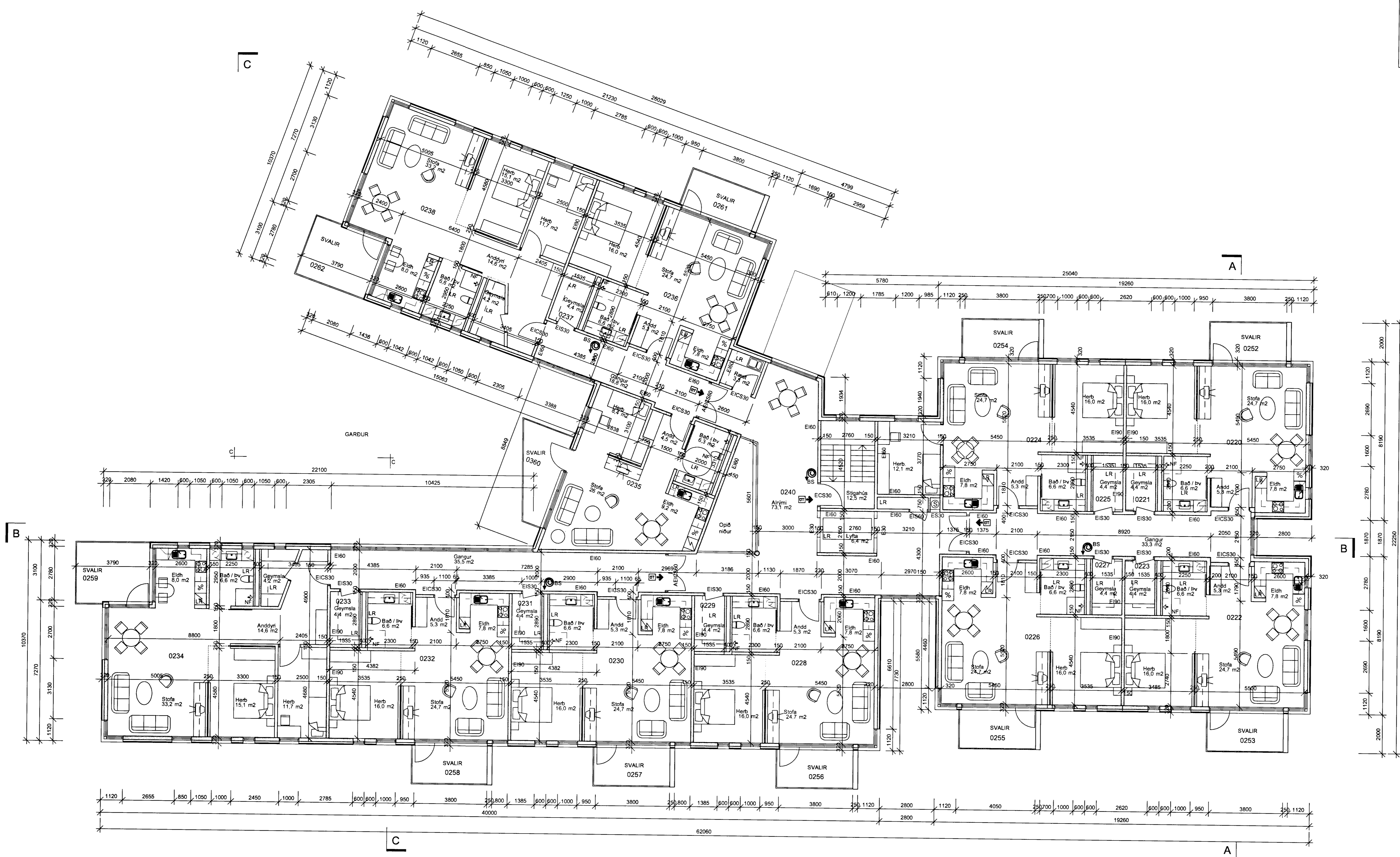
HÚS 2 - GRUNNMYND 2.HÆÐ 1:100
