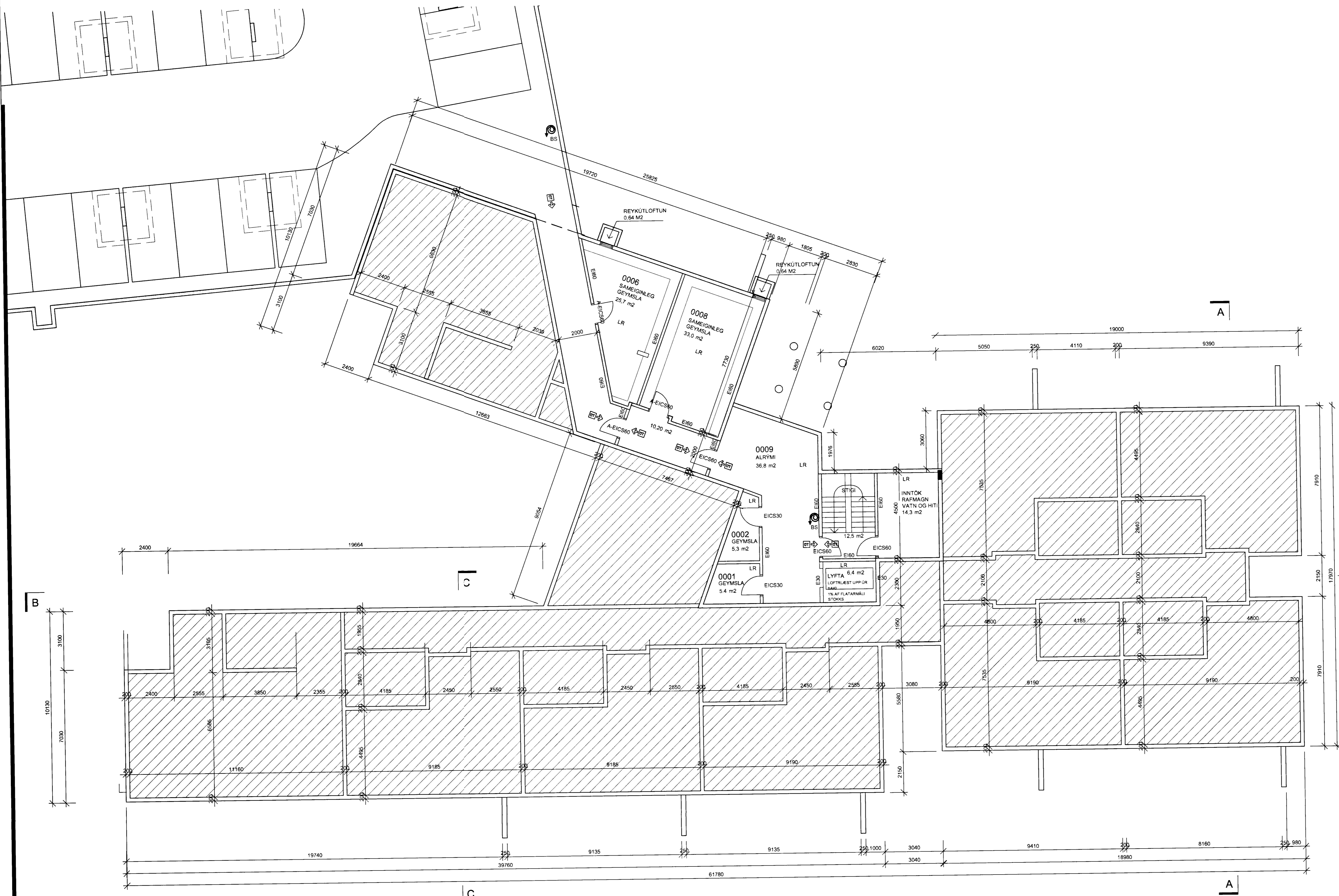
HÚS 1 - GRUNNMYND KJALLARA 1:100
