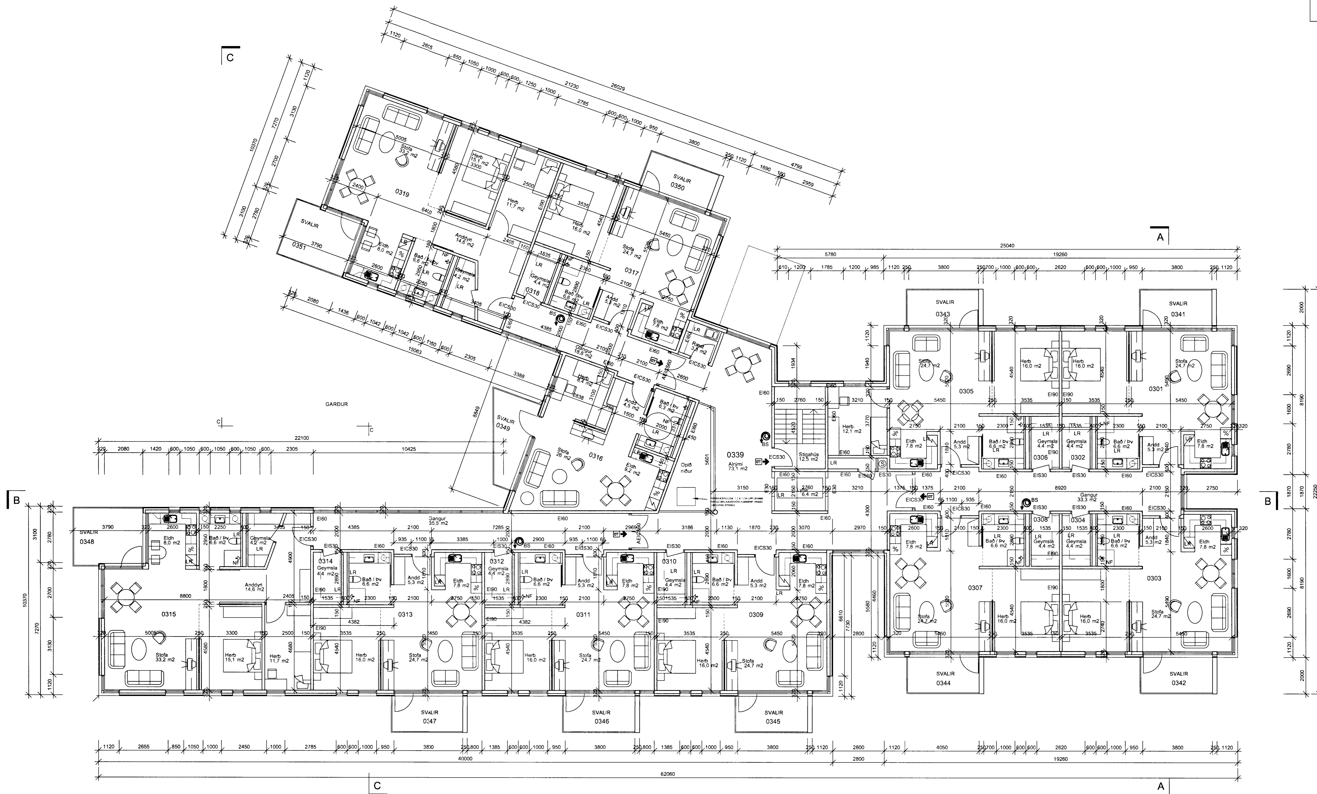
HÚS 1 - GRUNNMYND 3.HÆÐ 1:100
