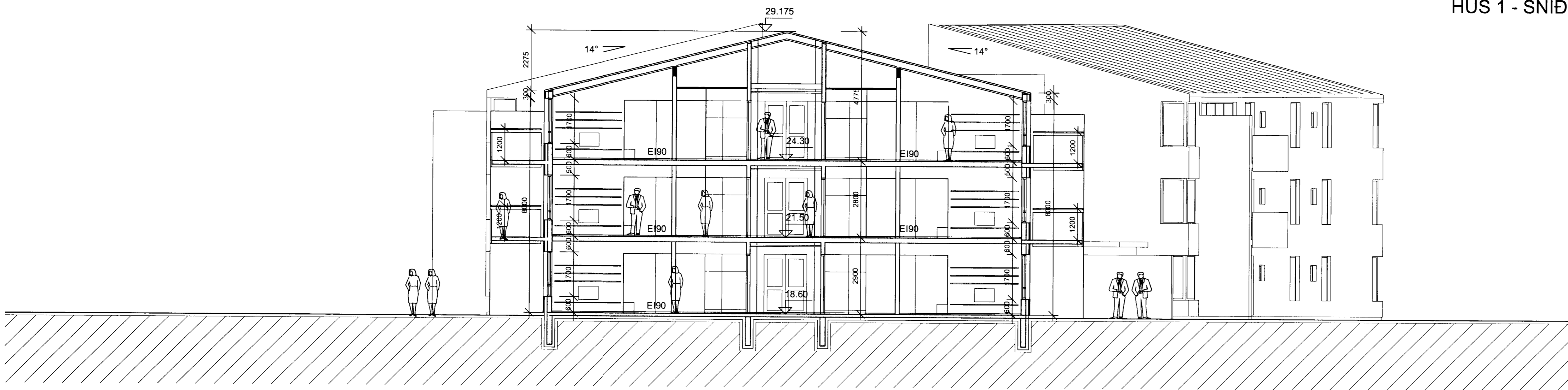
HÚS 1 - SNID A-A 1:100
