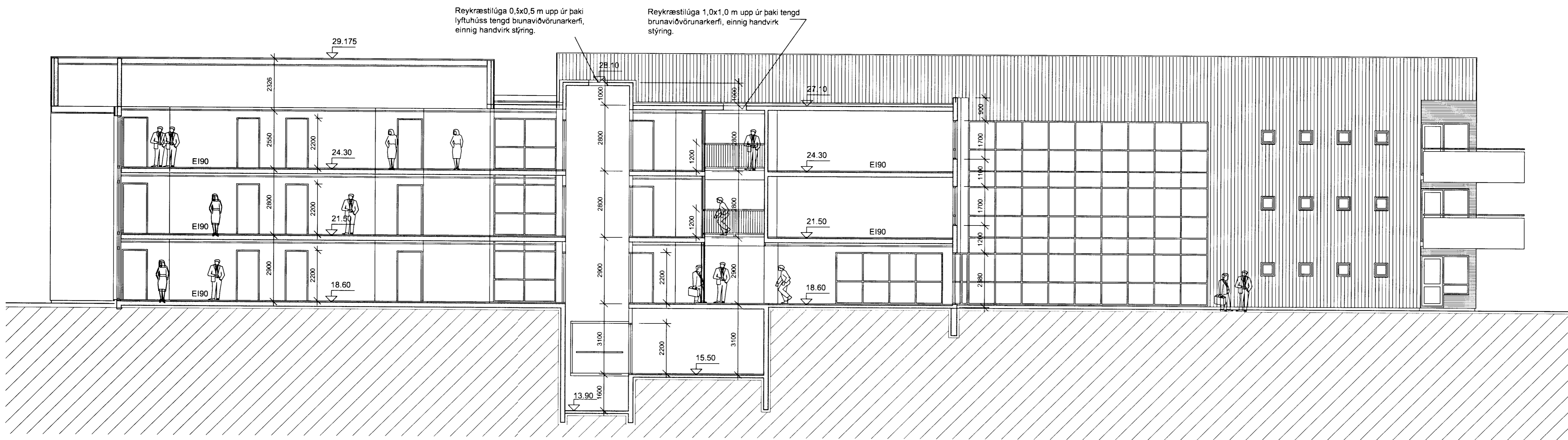
HÚS 1 - SNID B-B 1:100
