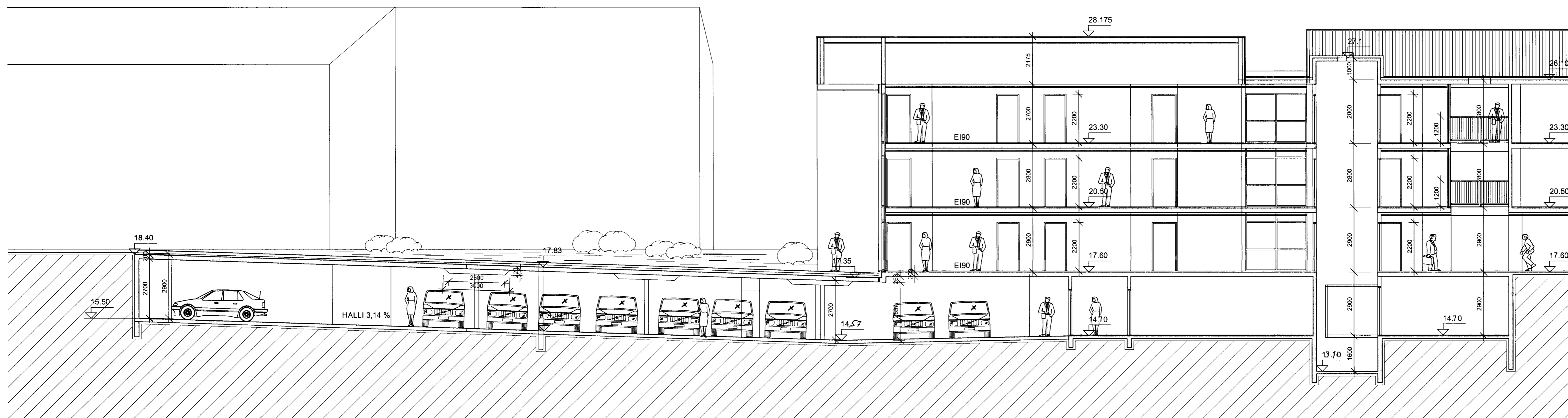
BÍLAKJALLARI - SNID H-H 1:100
