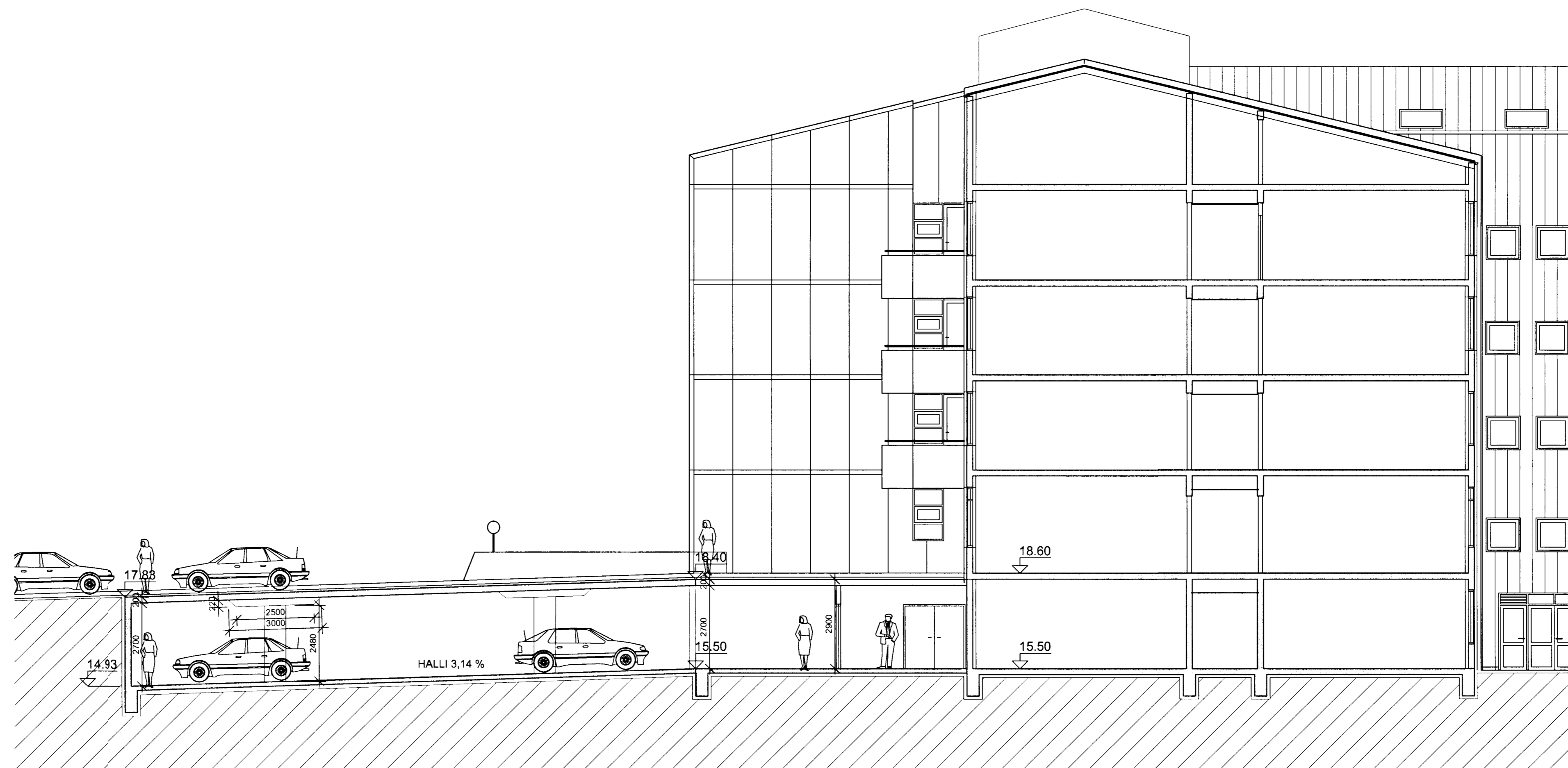
BÍLAKJALLARI - SNID G-G 1:100
