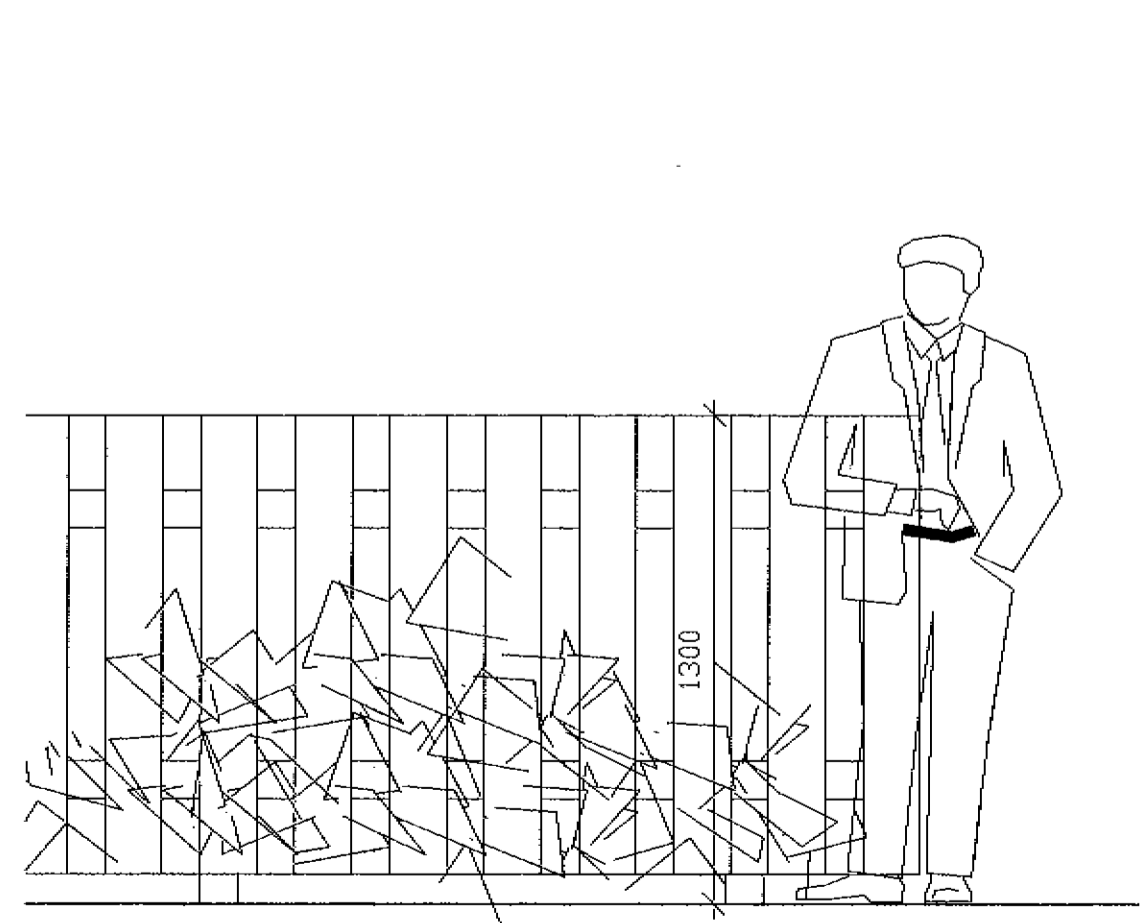
HLUTAÚTLIT GIRÐINGAR 1:20 VIÐ VERANDIR
