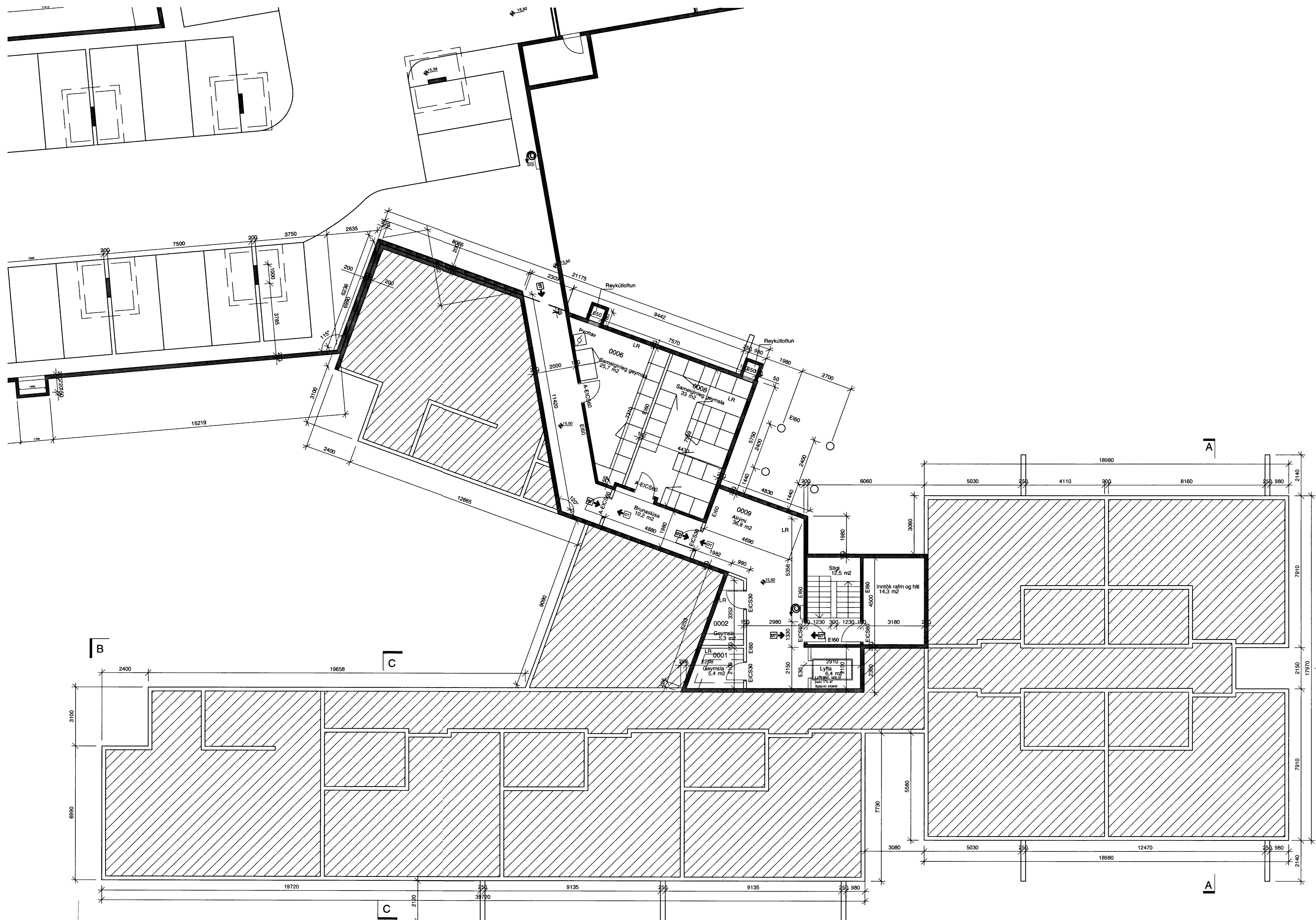
GRUNNMYND KJALLARA 1:100
