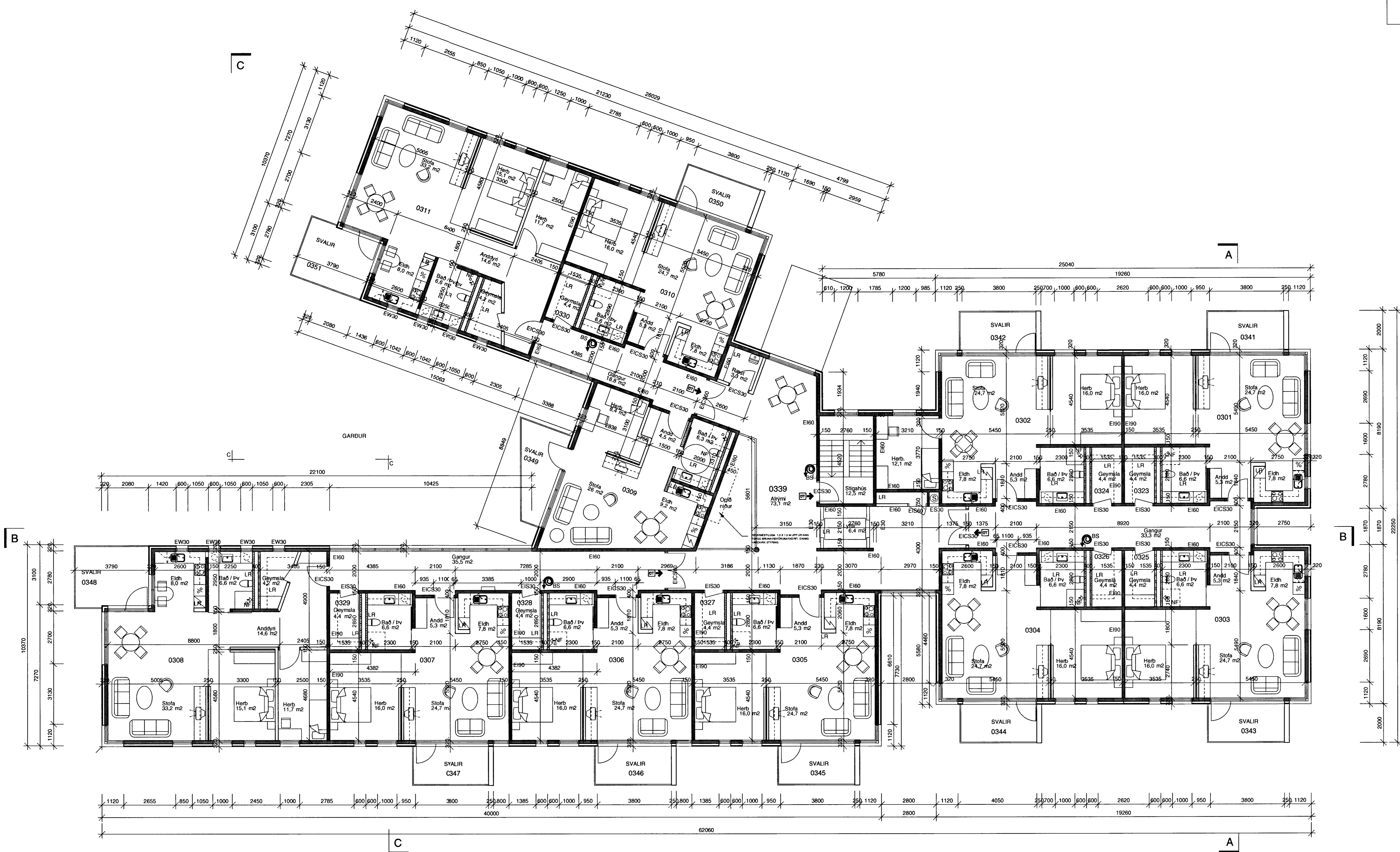
GRUNNMYND 3.HÆÐ 1:100
