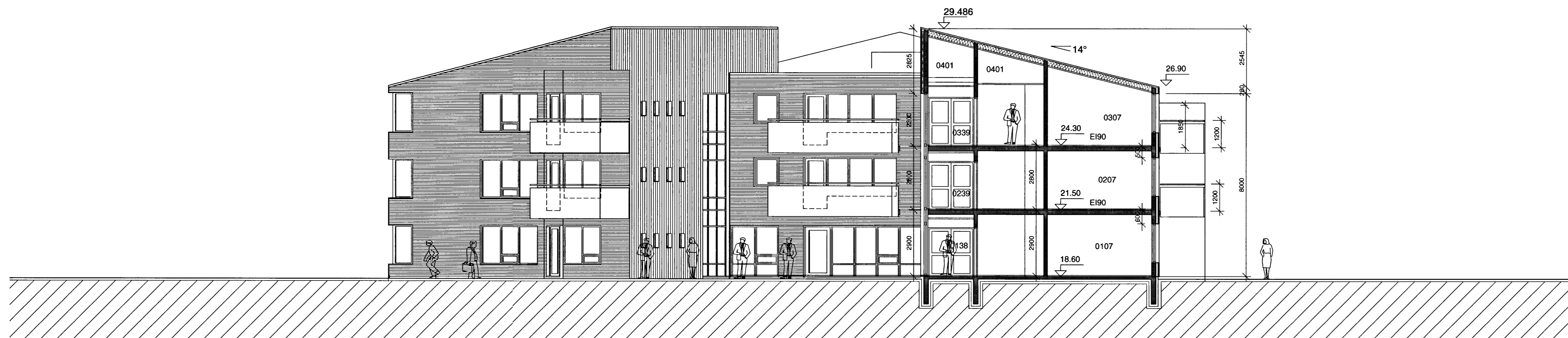
HRAUNVANGUR 1 SNID C-C 1:100
