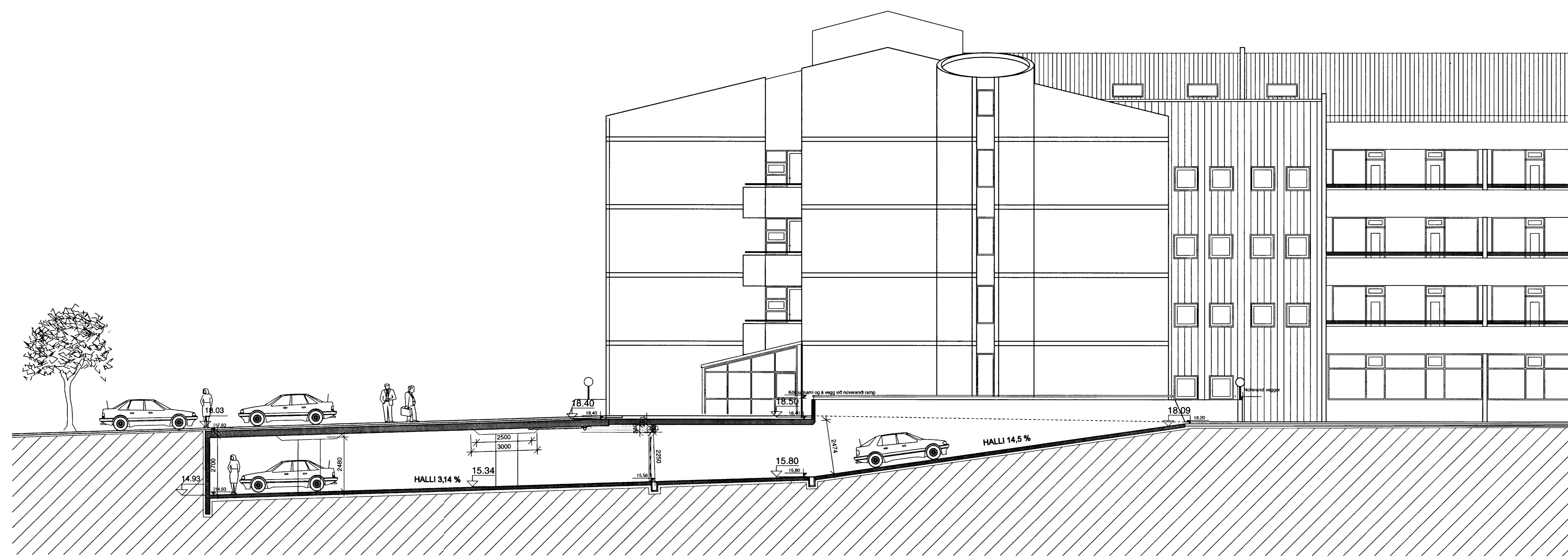
BÍLAKJALLARI SNÍÐ I-I 1:100
