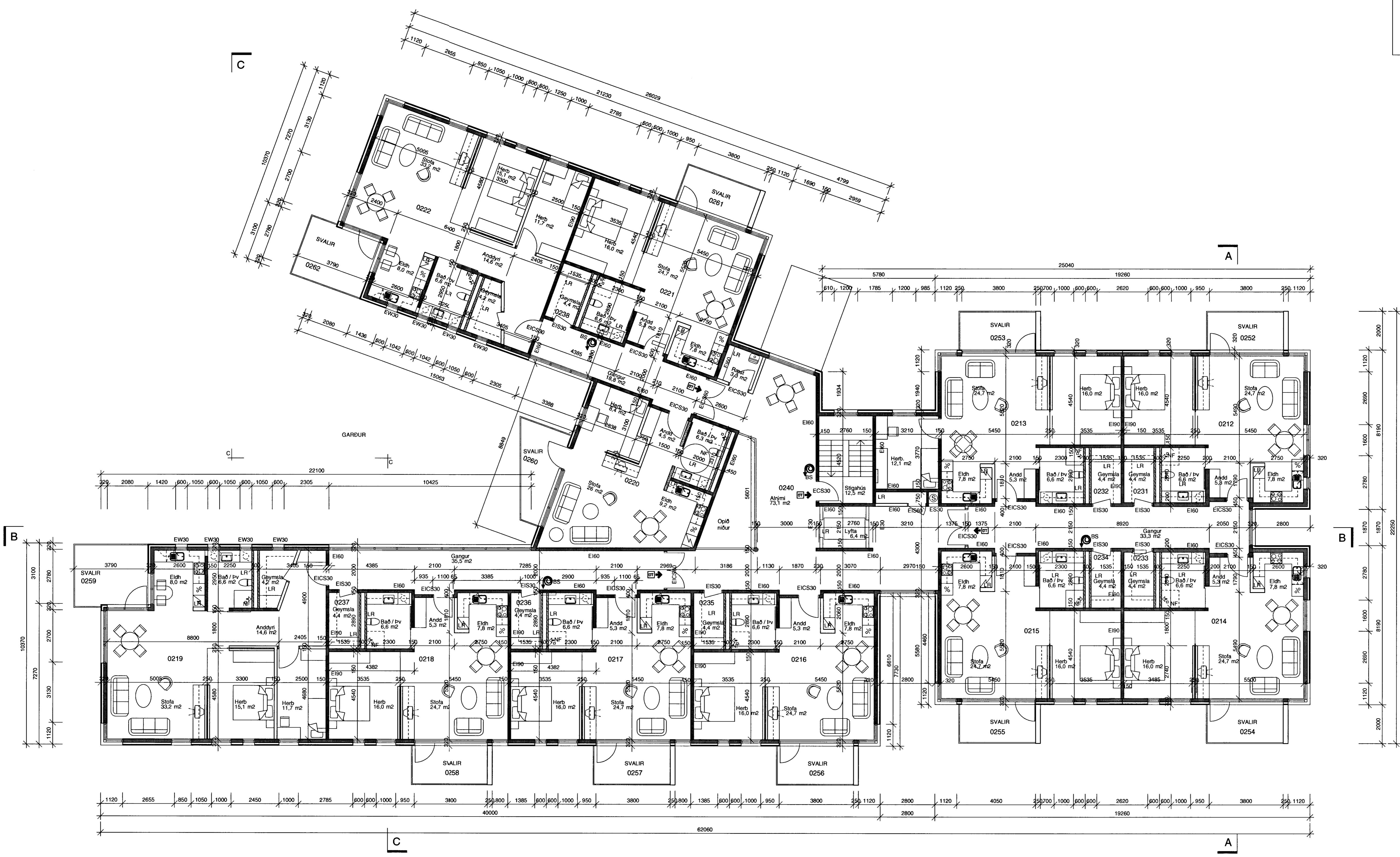
GRUNNMYND 2.HÆÐ 1:100
