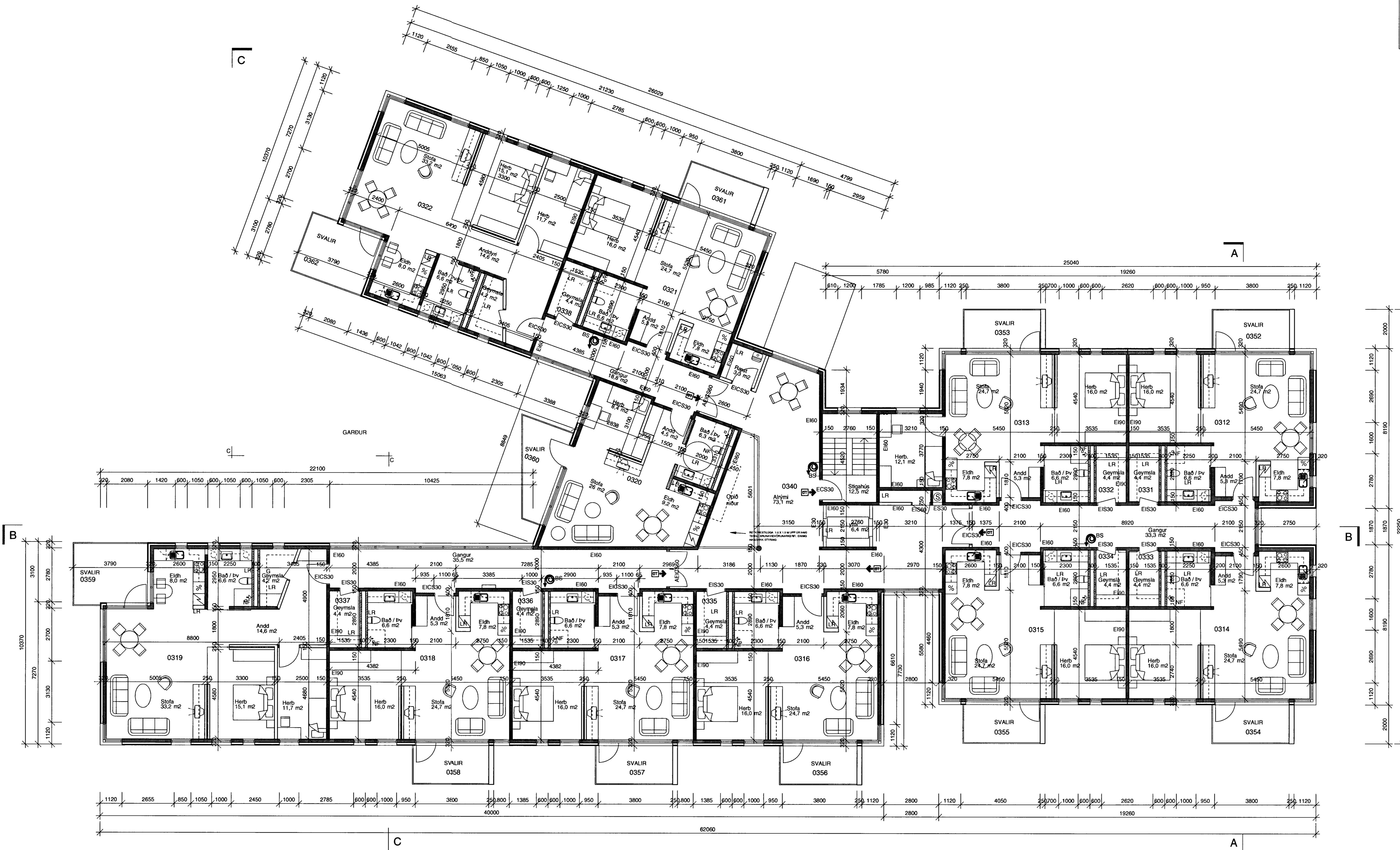
GRUNNMYND 3.HÆÐ 1:100
