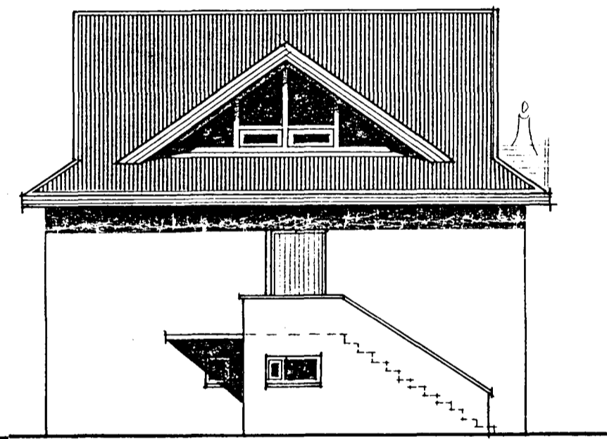
NORD - AUSTUR M = 1:100
