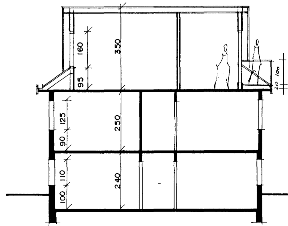
SNEIÐING B - B. M = 1:100
