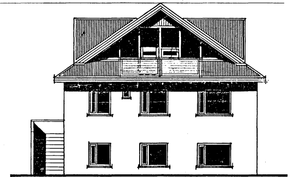
NORD - VESTUR M = 1:100
