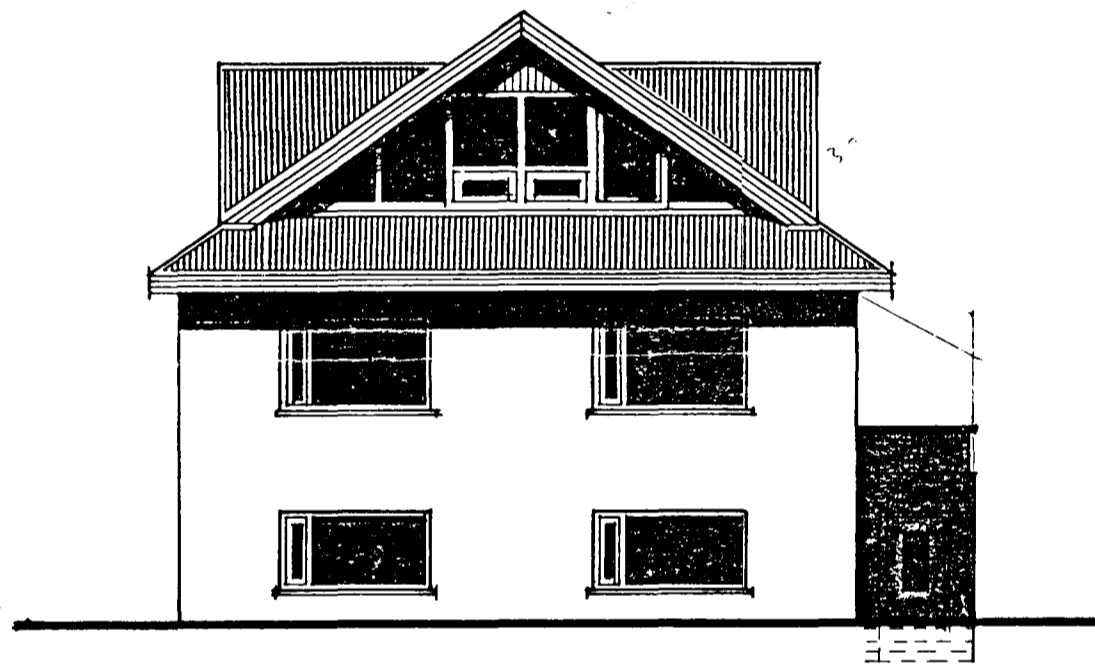
SUD - AUSTUR M = 1:100
