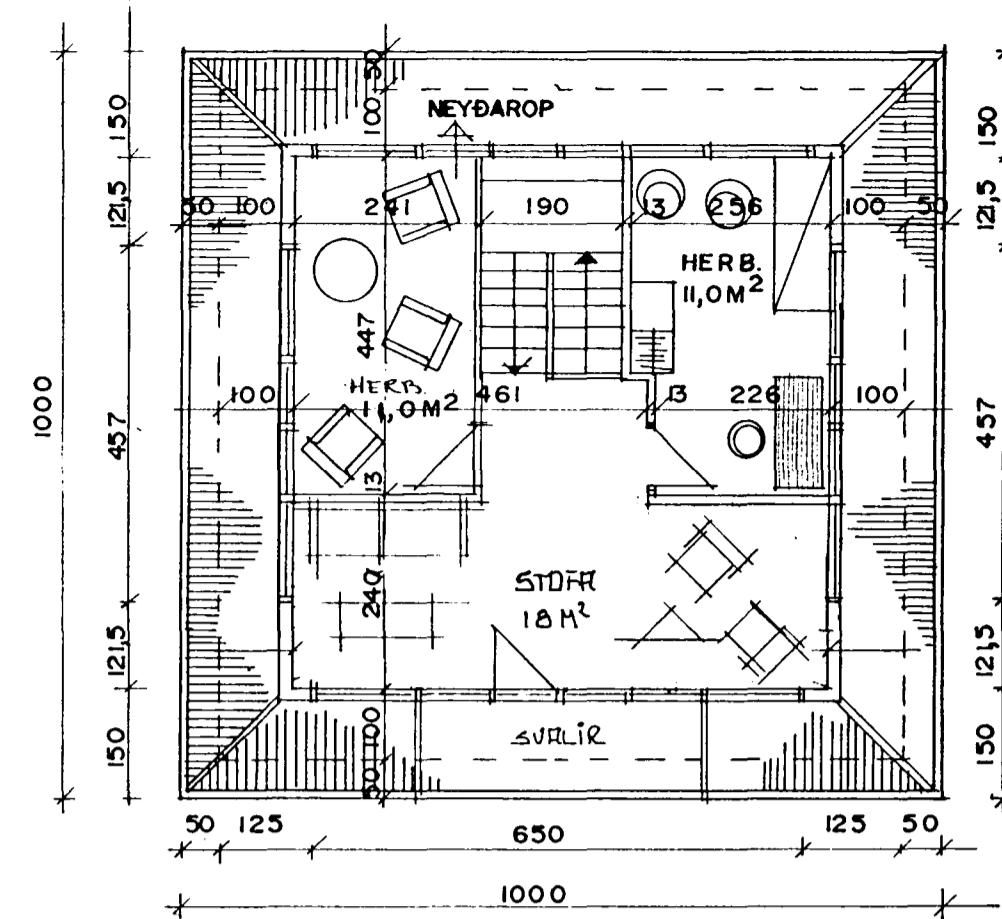
GRUNNMYND RISHÆÐAR M = 1:100
