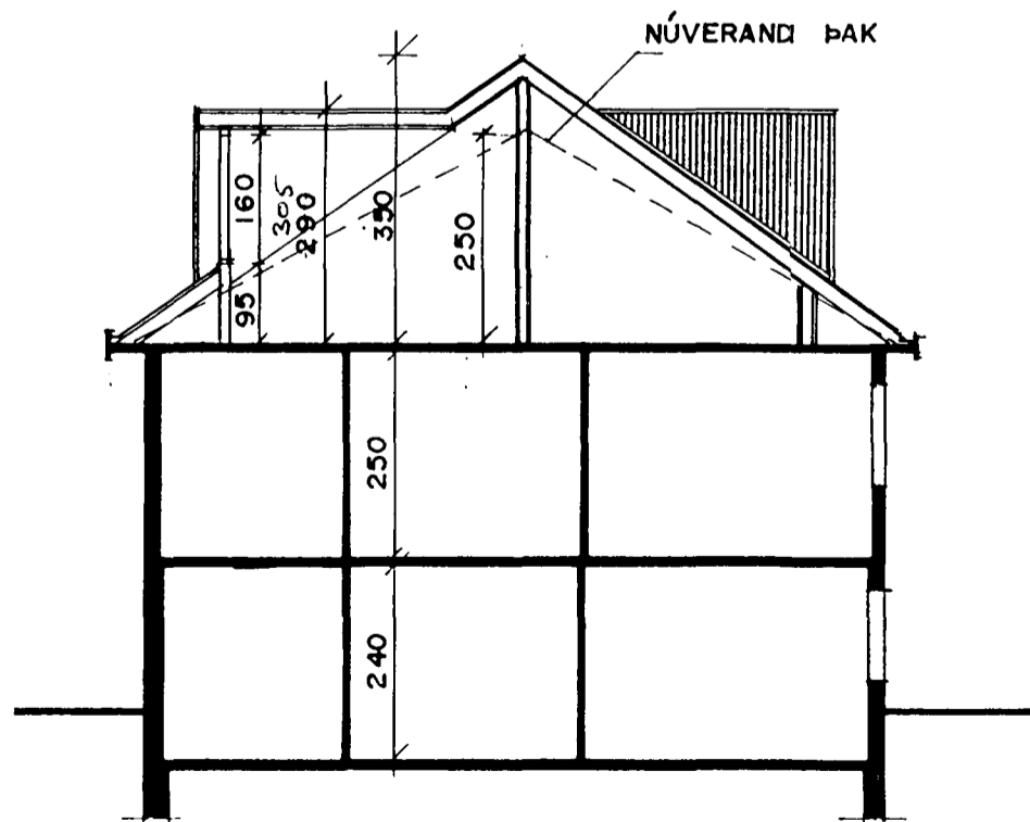
SNEIÐING A - A. M = 1:100
