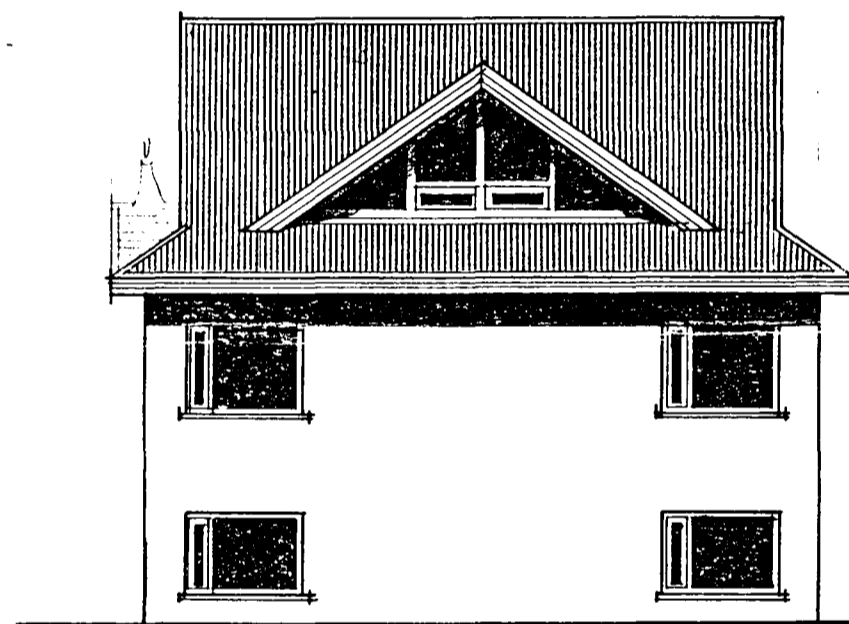
SUD - VESTUR M = 1:100
