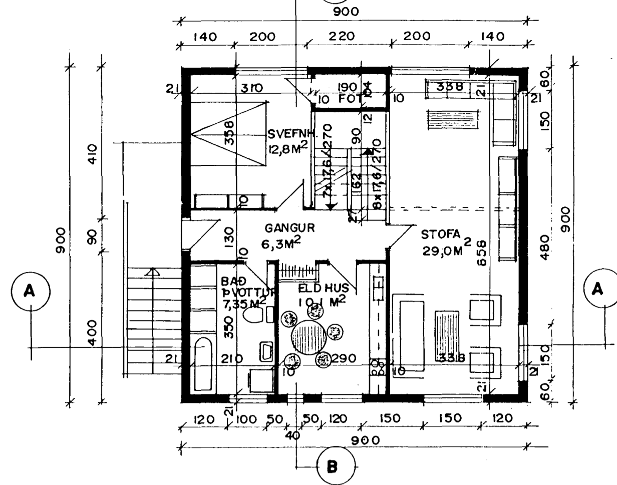
GRUNNMYND I. HÆÐAR. M = 1:100
