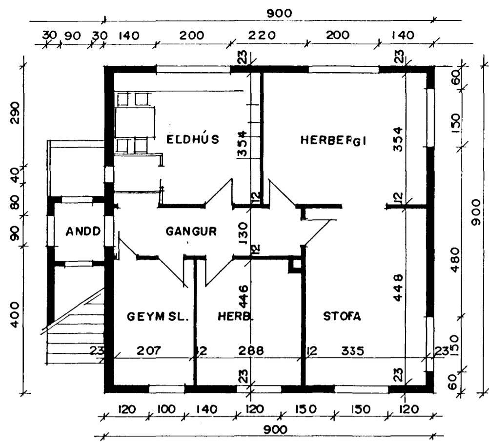
GRUNNMYND KJALLARA M = 1:100
