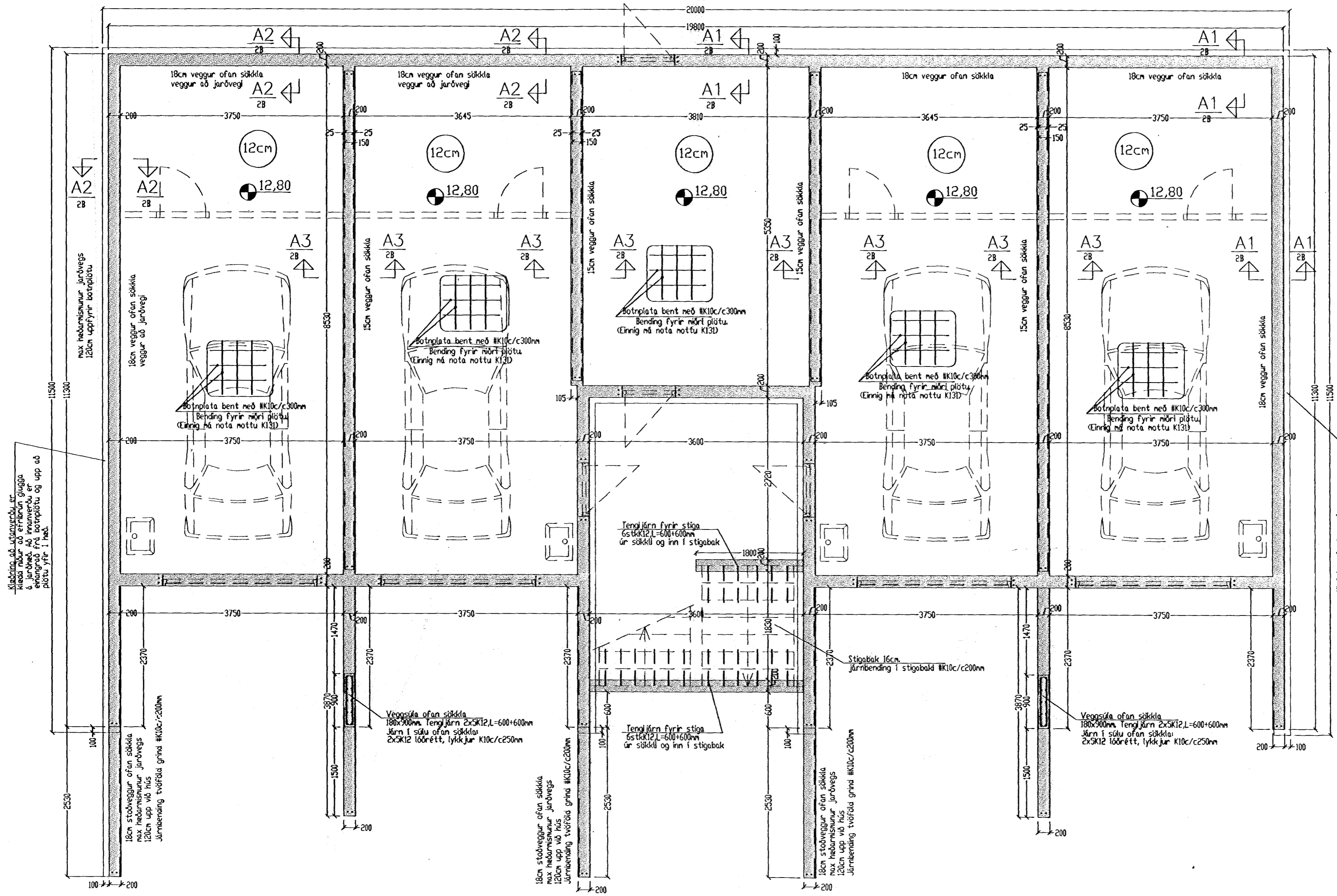
Grunnmynd sökkla 1:50
