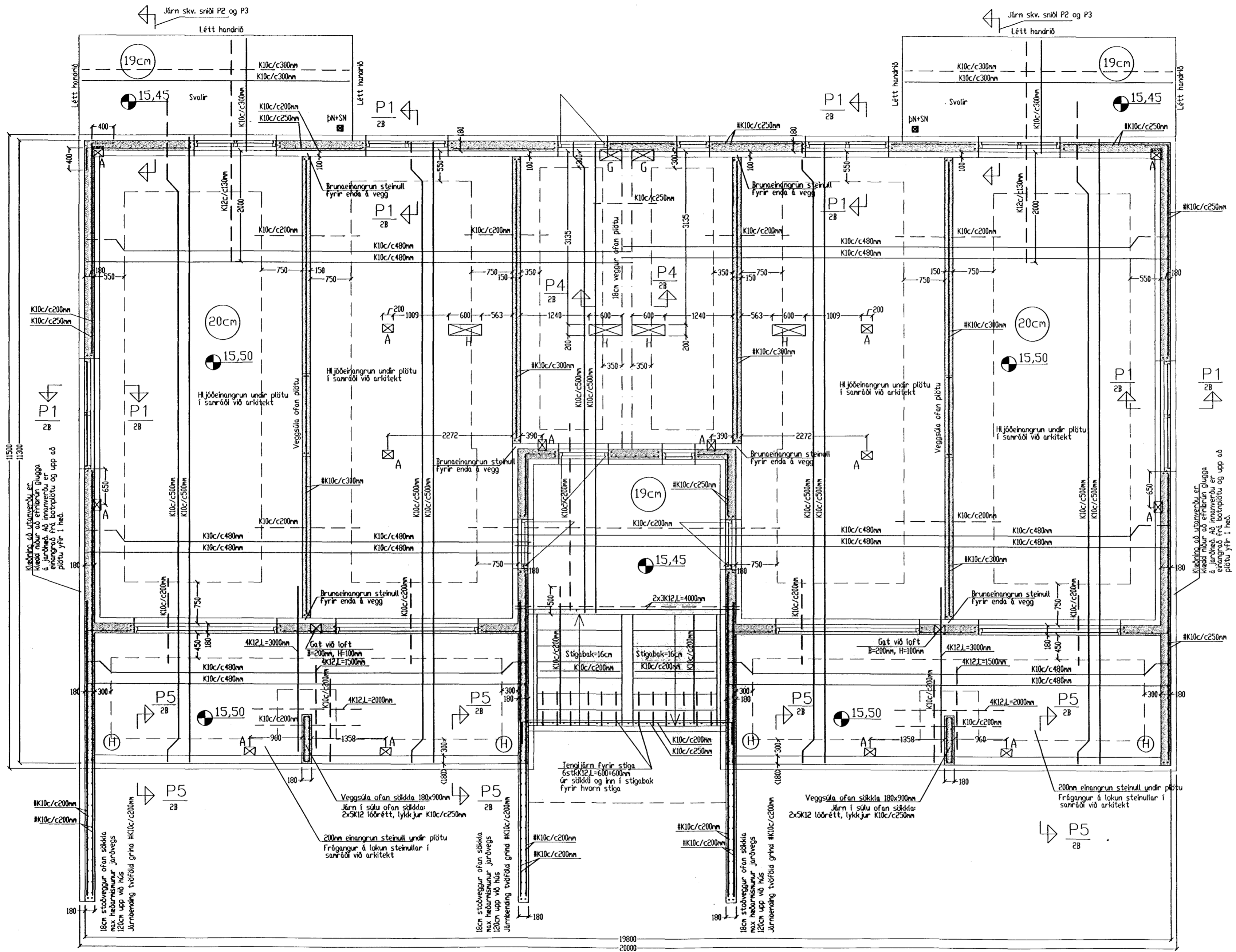
Grunnmynd plötu yfir jarðhæð 1:50
