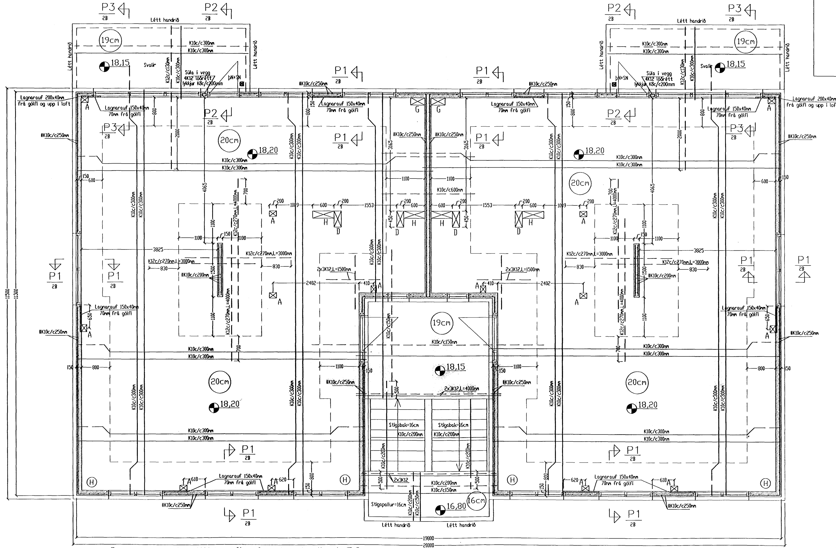
Grunnmynd plötu yfir fyrstu hæð 1:50
