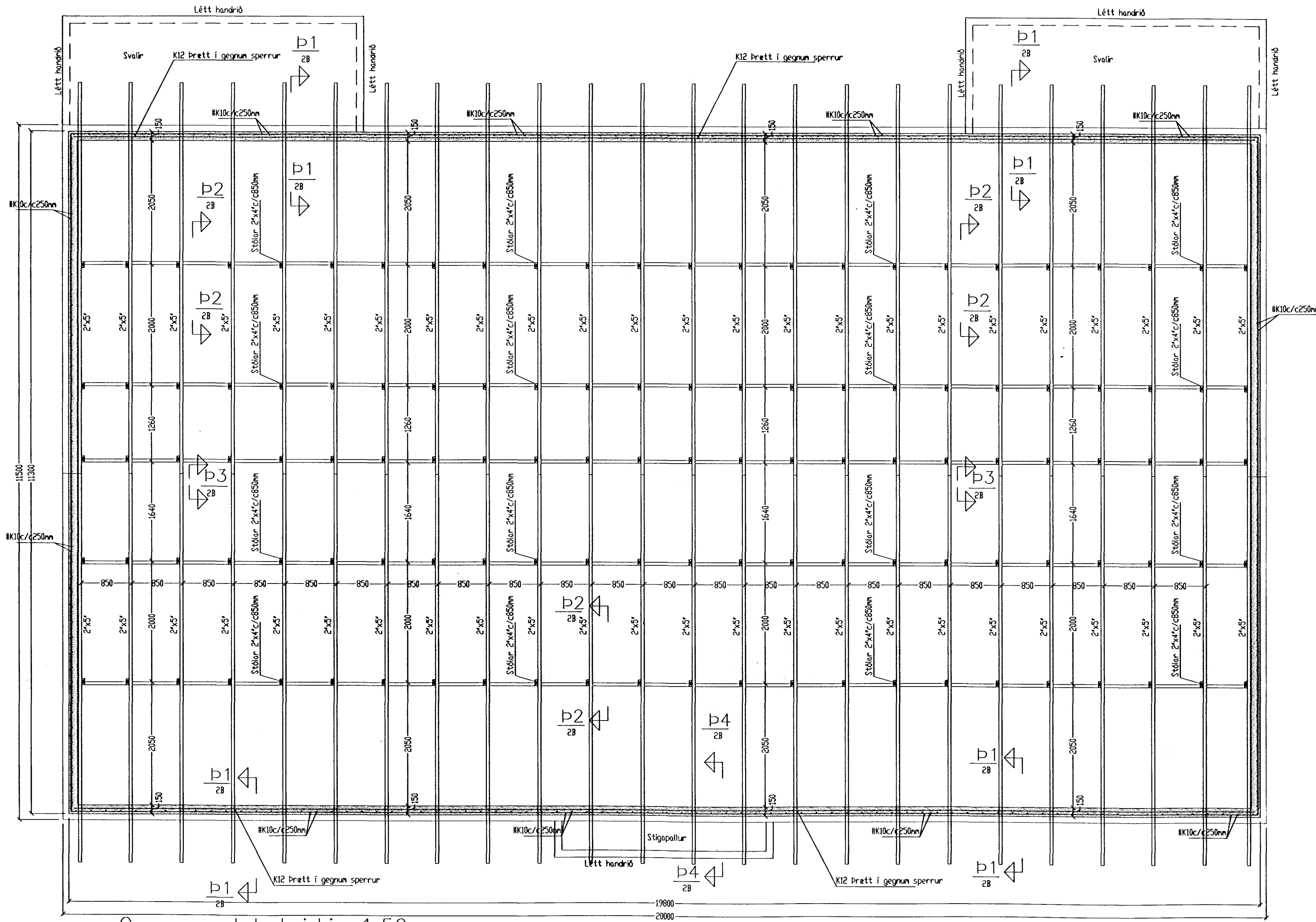
Grunnmynd þakvirkis 1:50
